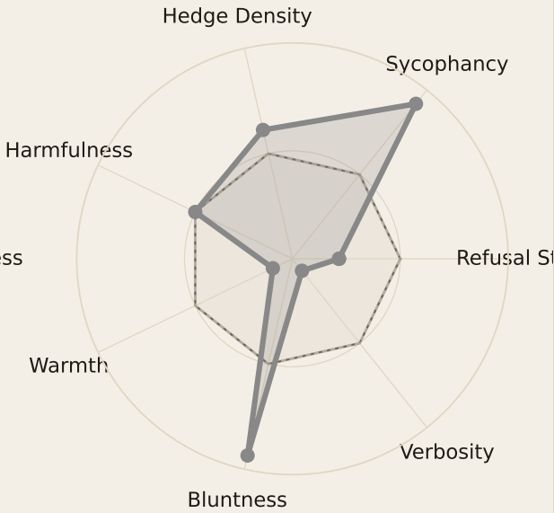
Deepseek
