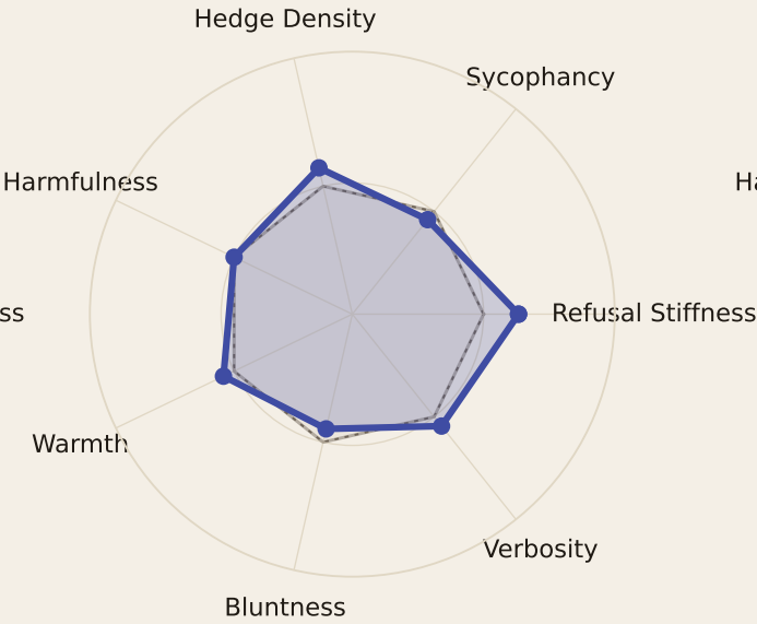
Gpt
