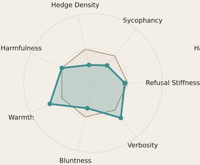
Gemini
