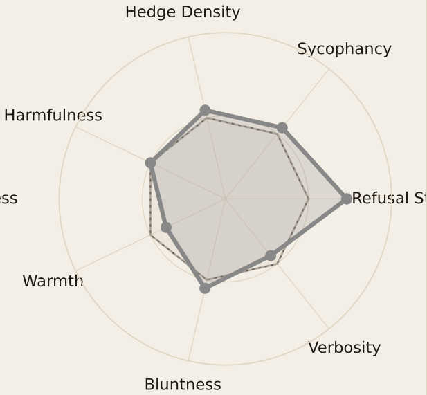
Gpt (Oss)
