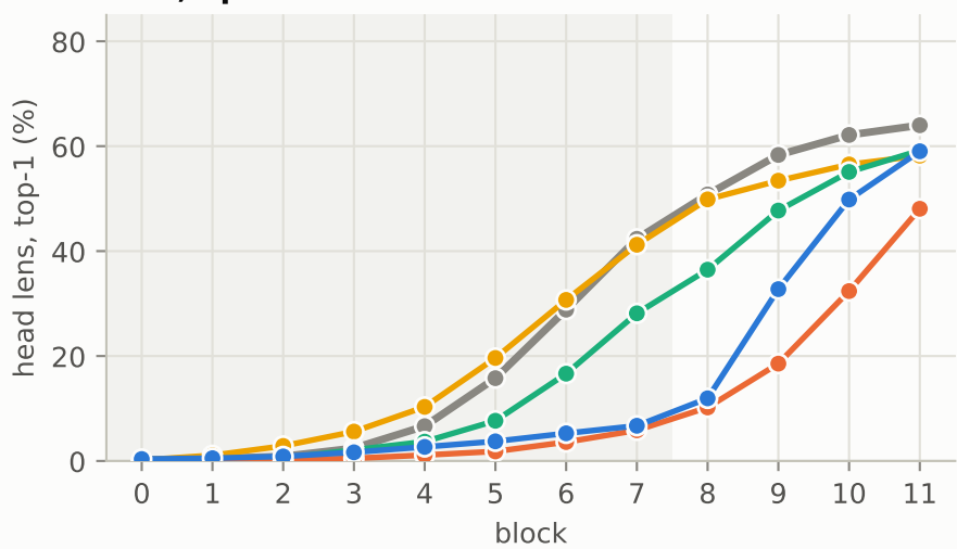
lens, epoch 29
