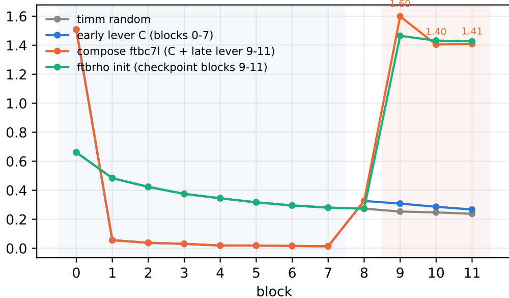
MLP write ratio \| \text{mlp}(x) \| / \| x \|
