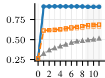
token cosine
