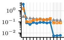
token cosine
