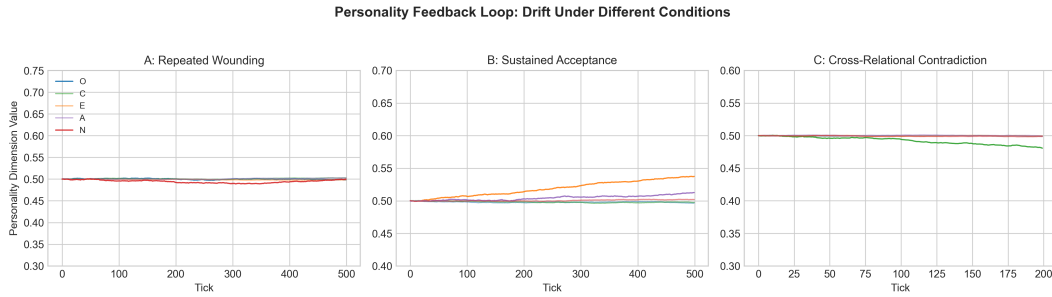
Figure 10: 人格反馈闭环验证。三种条件下人格向量的漂移轨迹：(A) 反复受伤 ( N \uparrow , O \downarrow )，(B) 持续接纳 ( E \uparrow , A \uparrow )，(C) 跨关系矛盾 ( C \downarrow )。漂移有界且由计算状态因果驱动。
