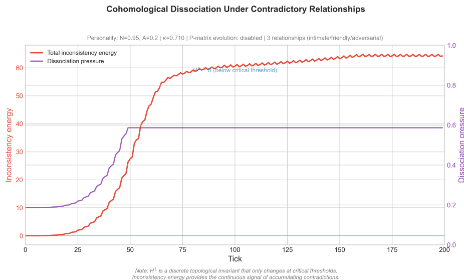
Figure 7: 200 tick 上同调解离检测。不一致性能量（S 曲线， 0 \rightarrow 65 ）和解离压力（ 0.19 \rightarrow 0.59 ）在矛盾事件下增长，而 H^1 保持为 0（满秩呈现矩阵阻止了真正的上同调阻碍）。
