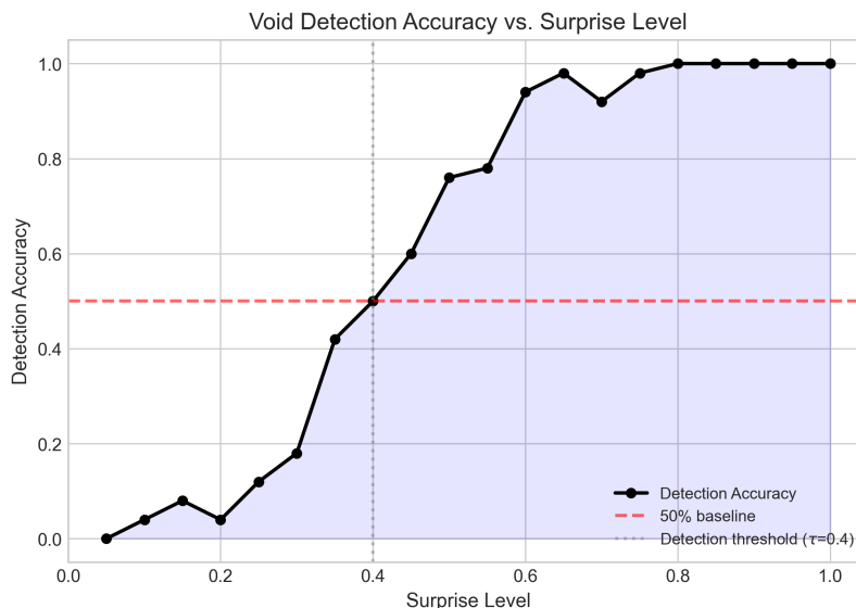
Figure 2: 空洞检测率 vs. 惊奇度水平。从 \sim 0\% 到 100\% 的平滑 sigmoid 过渡，每个水平 50 次试验，高斯噪声 \sigma = 0.15 。阴影区域显示检测阈值附近的过渡带。
