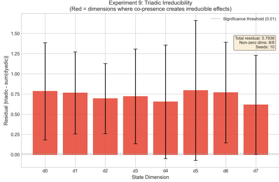
Figure 9: 8 个维度（10 个种子）的三元不可约性。所有维度显示显著重构残差（均值 0.62–0.79）；总残差 = 5.79，确认仅从成对数据不可获得的不可约三元信息。
