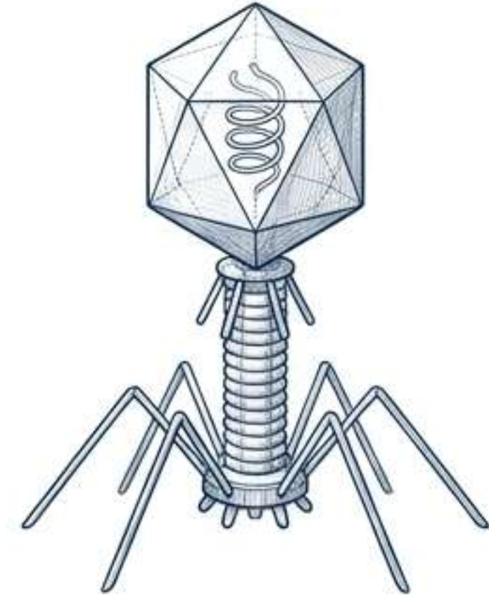
Symétrie Complexe
