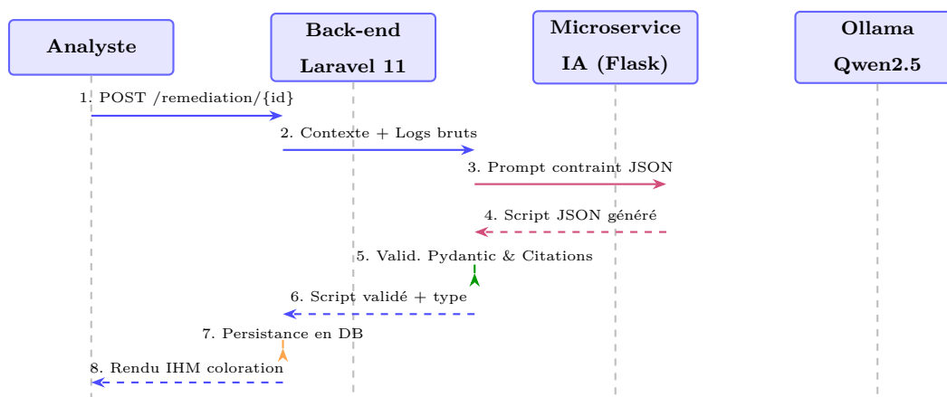
Figure 3.9 : Diagramme de Séquence – Génération de Remediation-as-Code Assistée par IA
