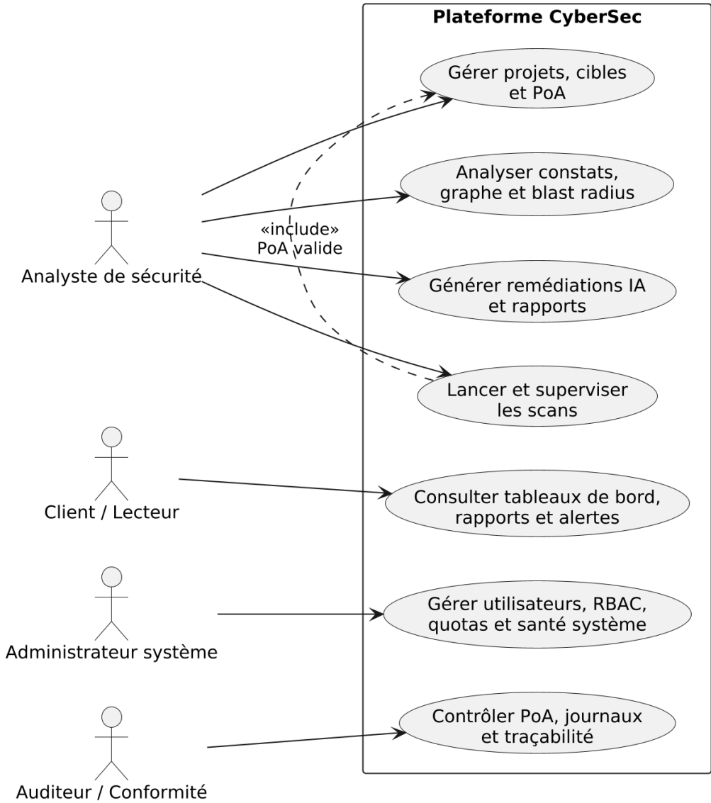
Figure 3.1 : Diagramme Global des Cas d’Utilisation – Acteurs et Fonctionnalités Clés
