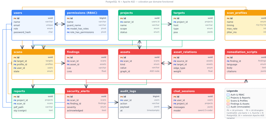
Figure 3.6 — Diagramme Entité-Association (14 tables)
