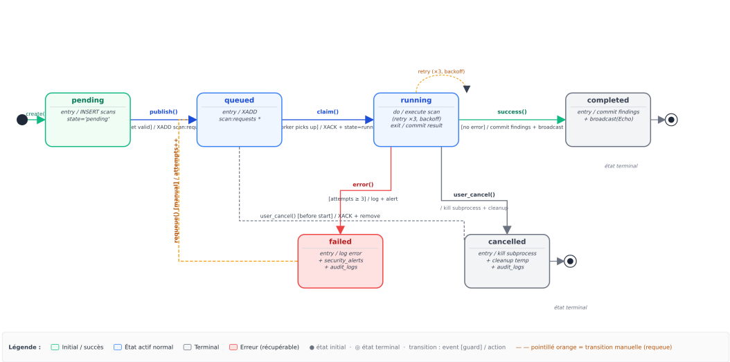
Figure 3.9 — Machine à états : cycle de vie d'une tâche de scan
