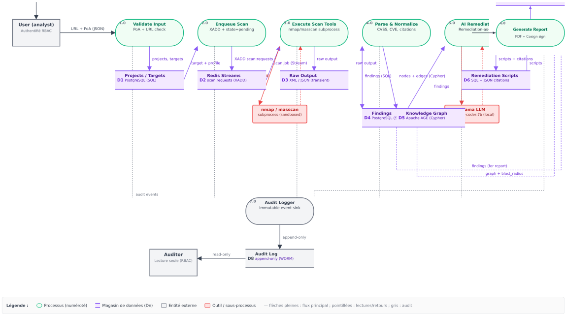
Figure 3.10 — Diagramme de flux de données (DFD) de la plateforme
