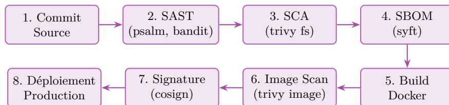
Figure 3.14 : Pipeline DevSecOps Automatisé – Chaîne de Sécurité Intégrée sous GitHub Actions
