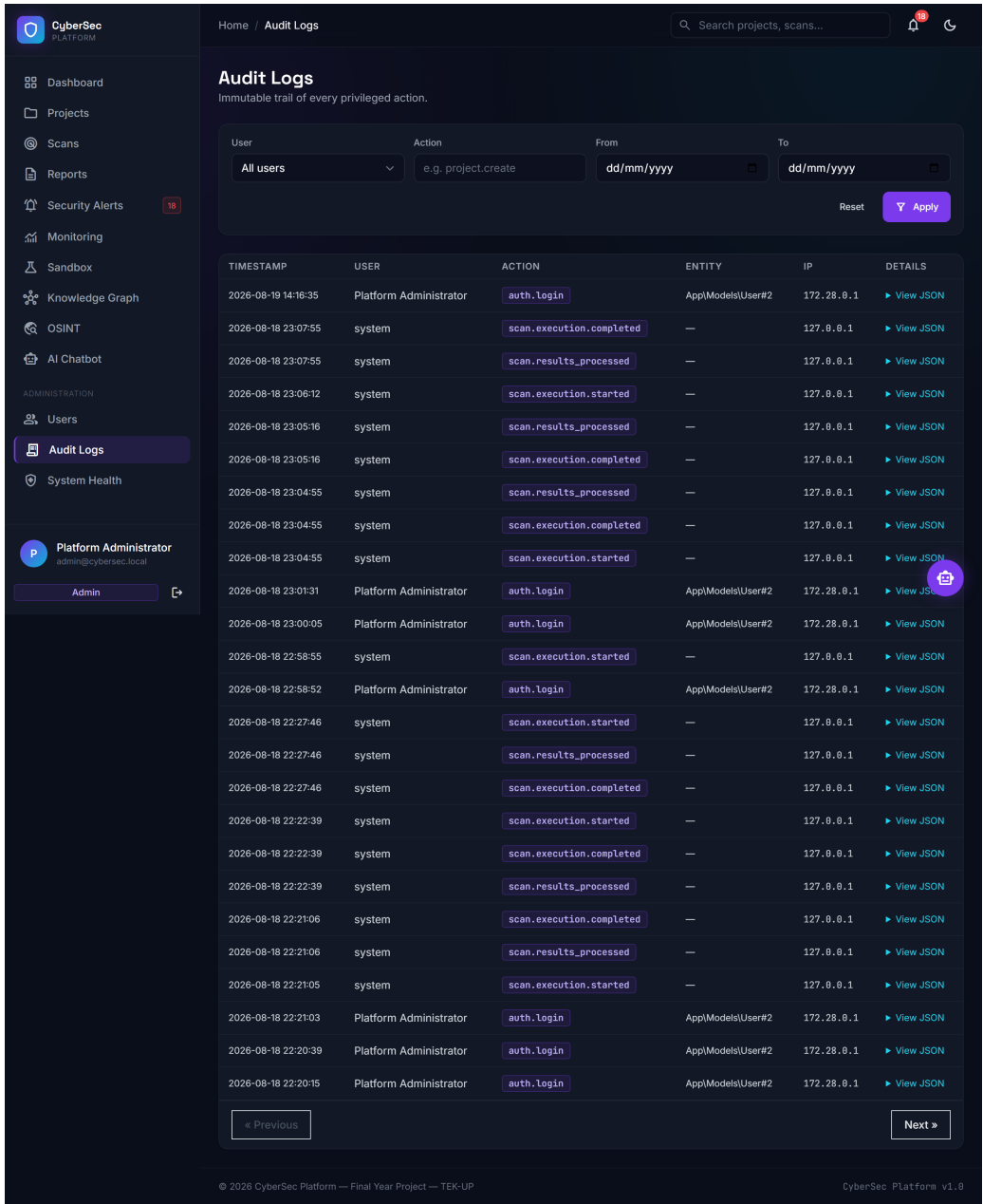
Figure 4.19 : Module de Journalisation d’Audit Immuable pour la Traçabilité des Événements
