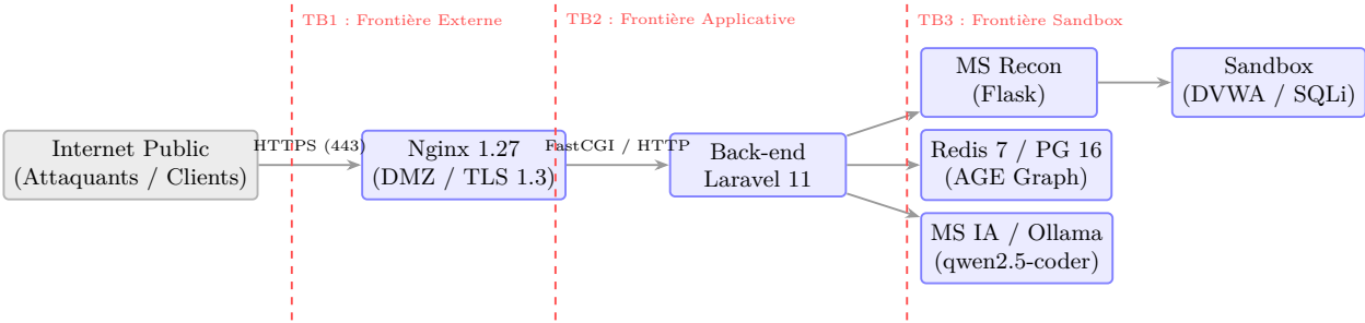
Figure 3.13 : Cartographie de la Surface d'Attaque et Frontières de Confiance (Trust Boundaries)
