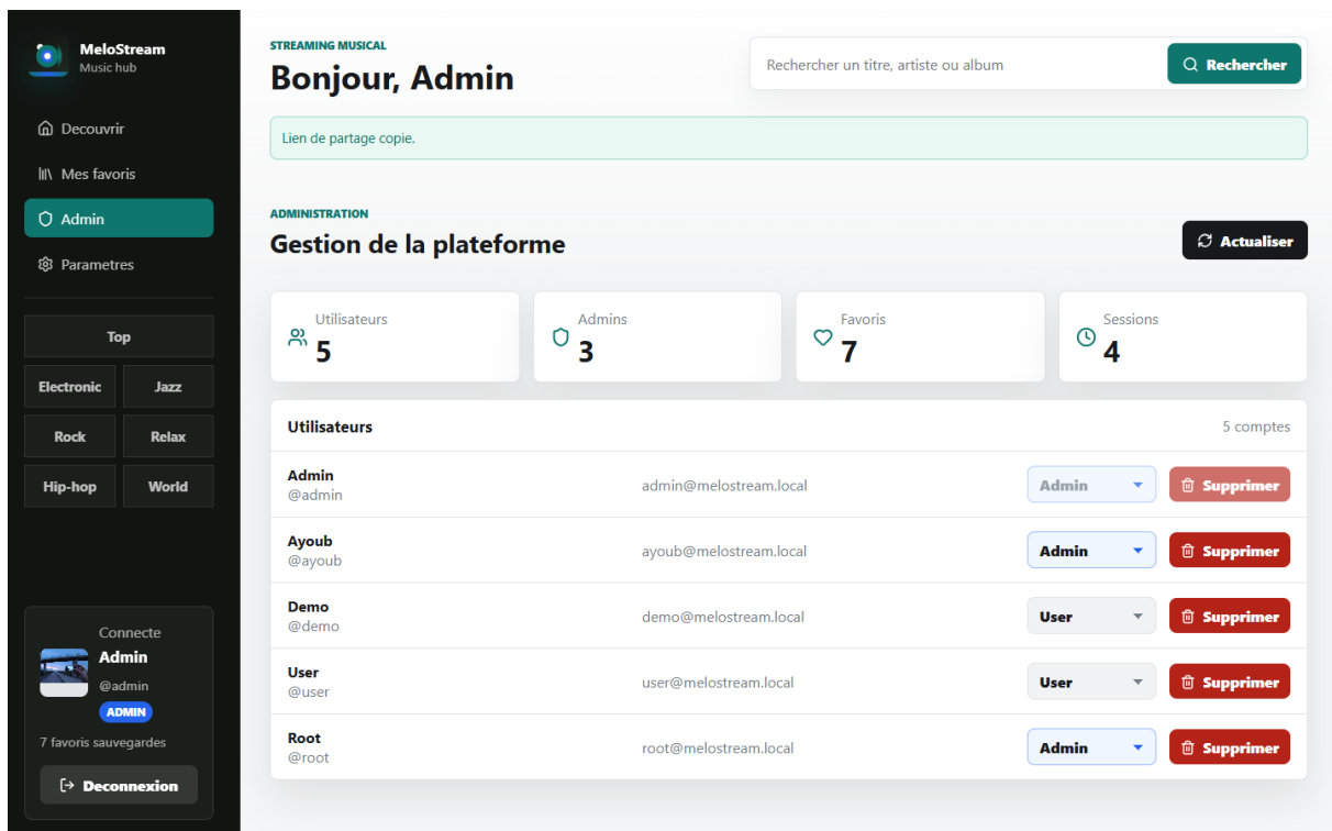
FIGURE 4.9 – Interface d'administration
