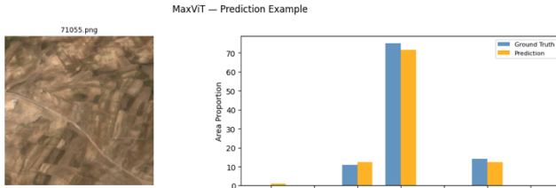
Fig. 1. MaxViT Prediction Example
