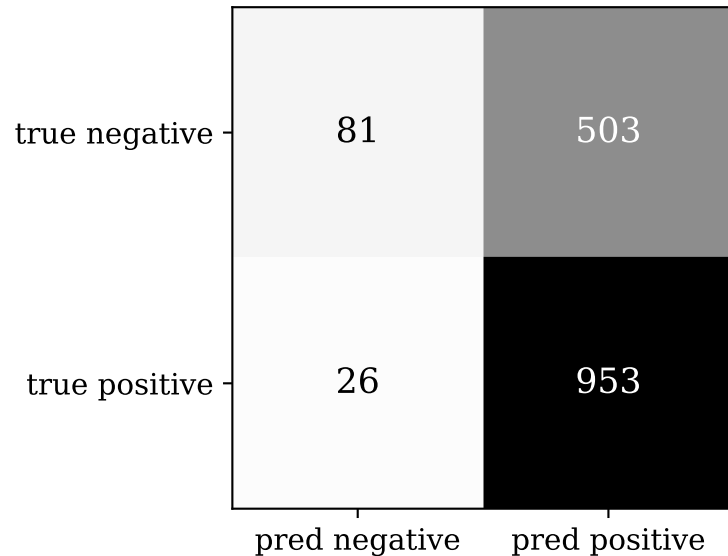
Confusion matrix @ 46 °C (best F1 = 0.78)
