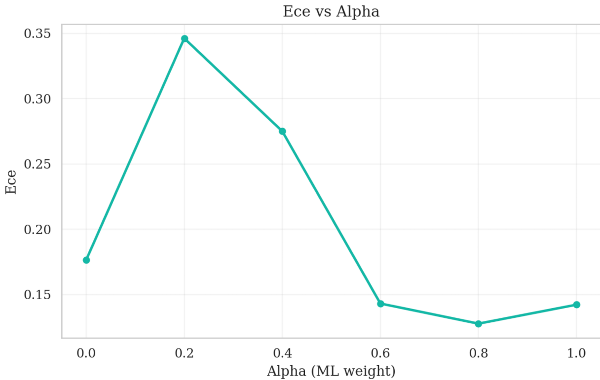
ece vs alpha
