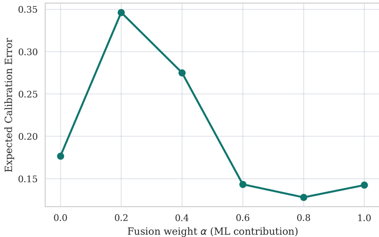
ece vs alpha
