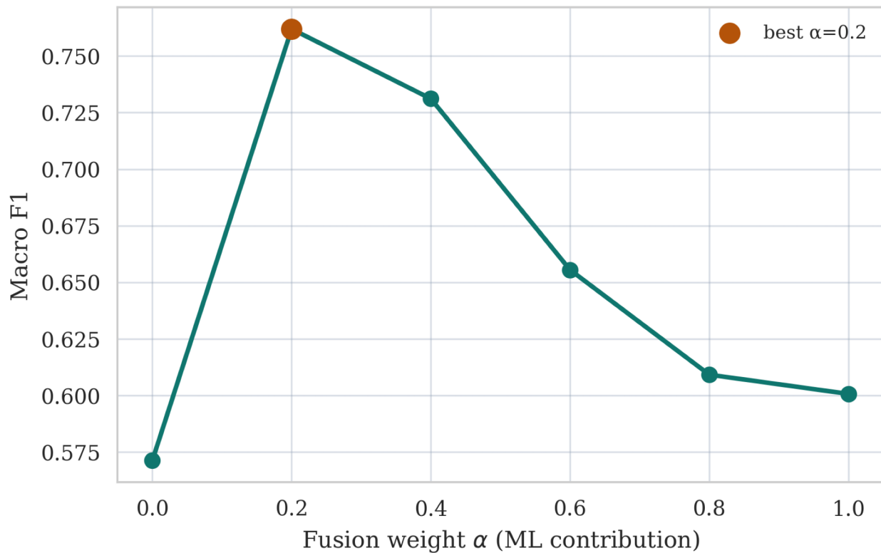
macro f1 vs alpha
