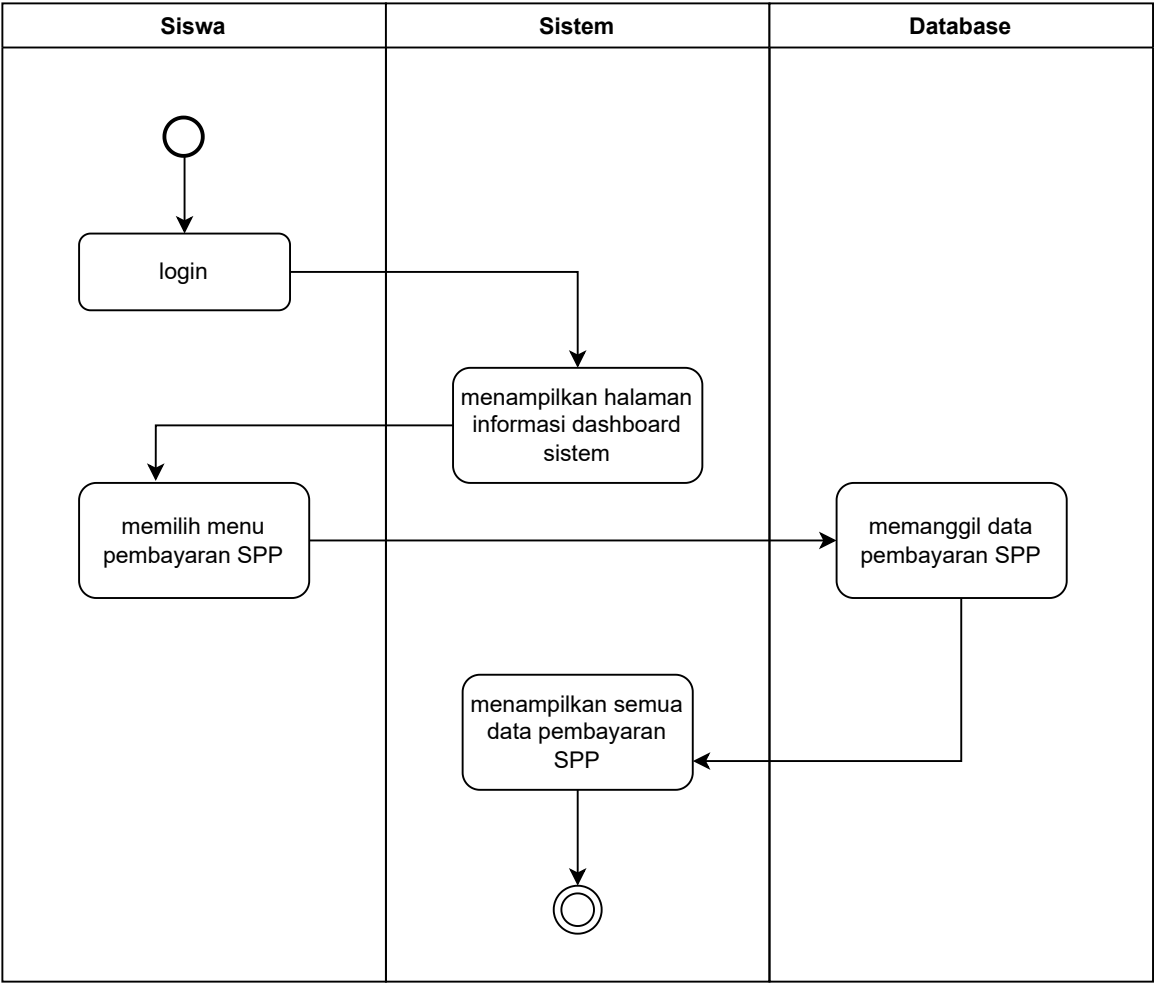
activity diagram melihat pembayaran SPP
