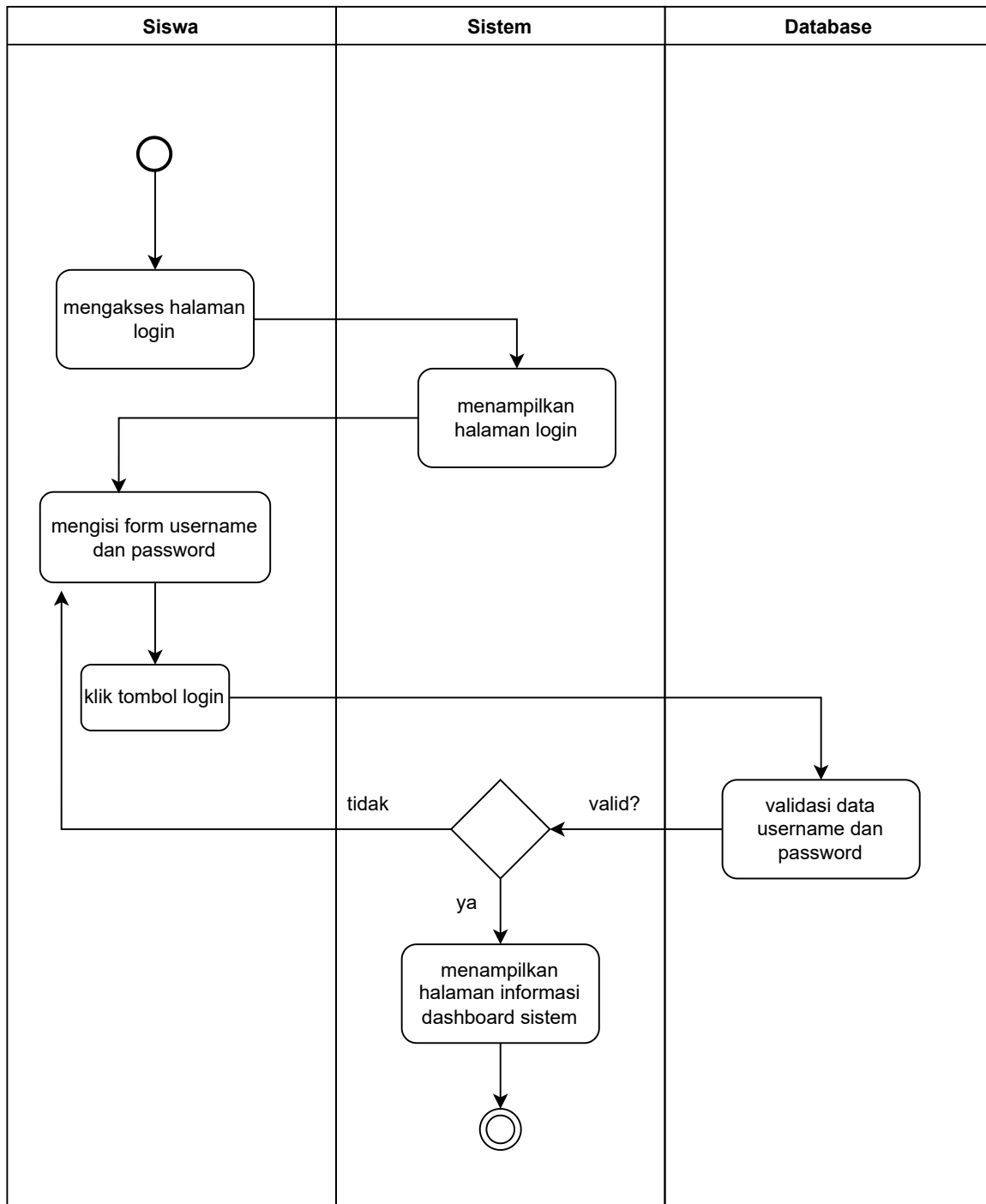
activity diagram melihat informasi dashboard sistem siswa
