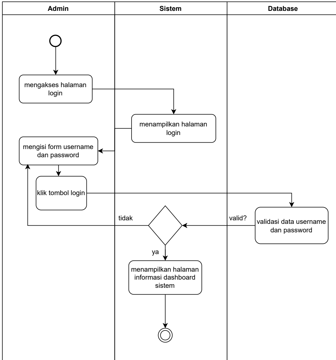
Activity Diagram Login dan Melihat Informasi Dashboard Sistem
