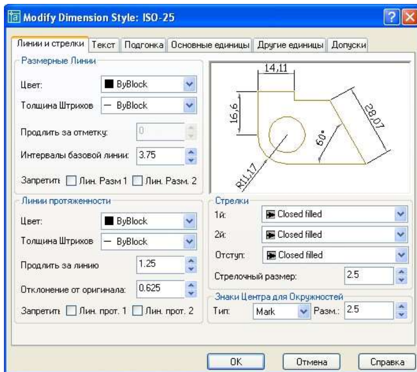
5.5-rasm. O'lcham chiziq va strelkalarini o'zgartirish dialog oynasi
