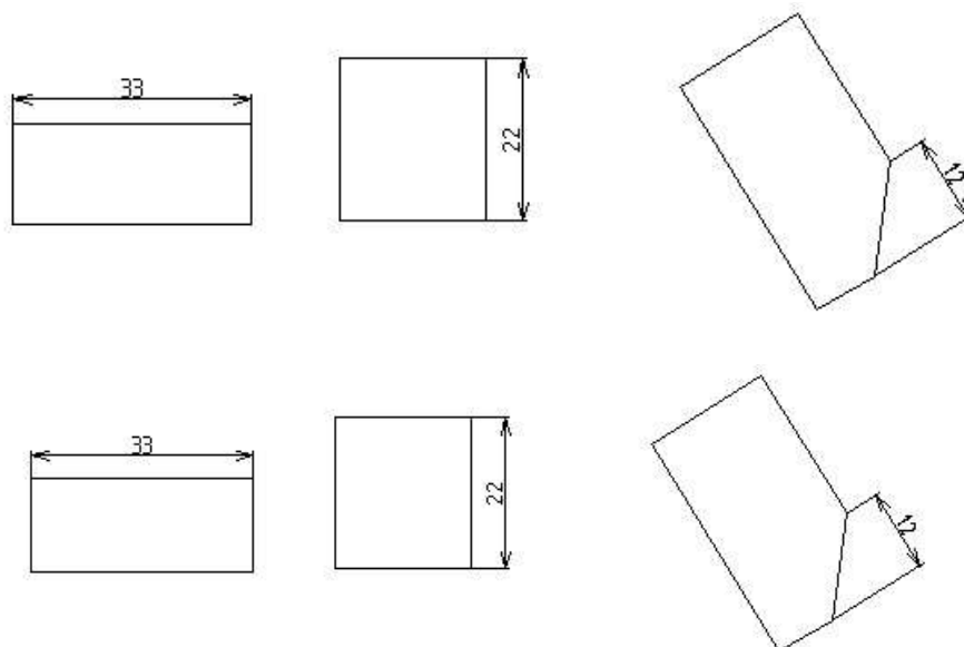
5.10-rasm. Chiziqli o'lchamlarni qo'yish
