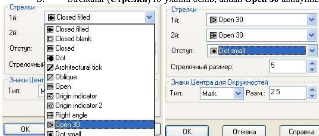
5.5-rasm. O'lcham chiziq va strelkalarini o'zgartirish dialog oynasi
