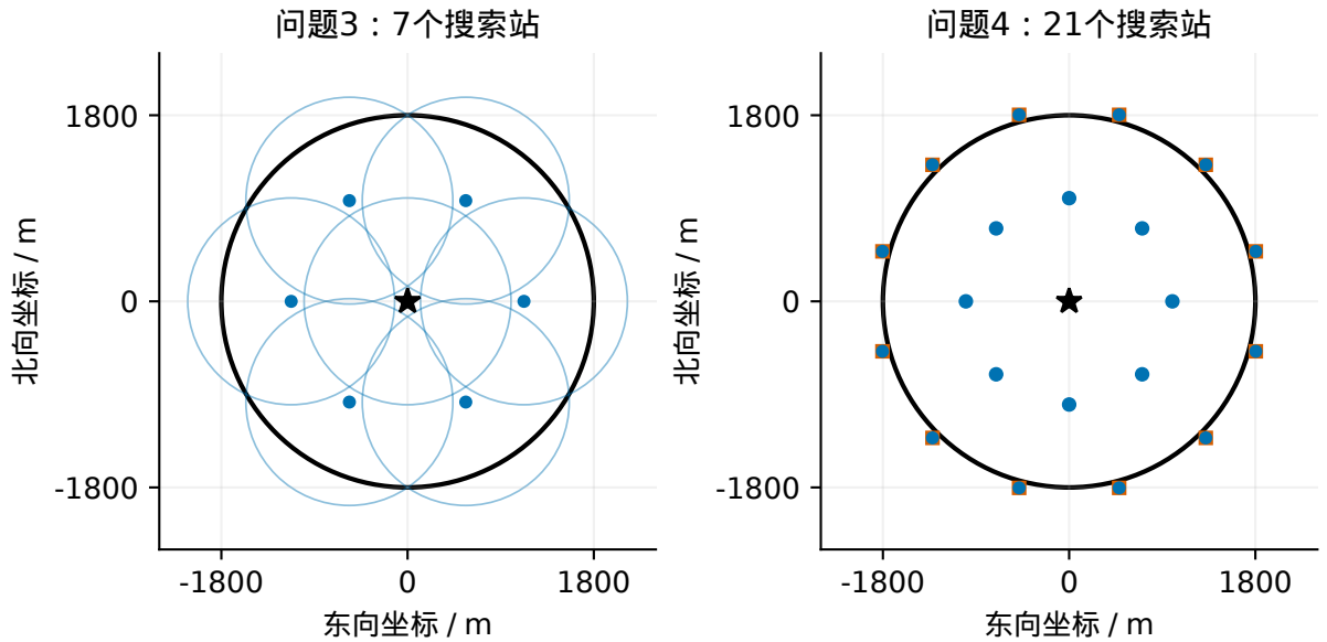
图 3 搜索站布局。左图的浅色圆为 1000 米接收圆，覆盖 1800 米源域；右图为问题四的 21 站，其中外环半径 1868 米。点集只提供初始覆盖结构，实际访问顺序随任务状态调整。
