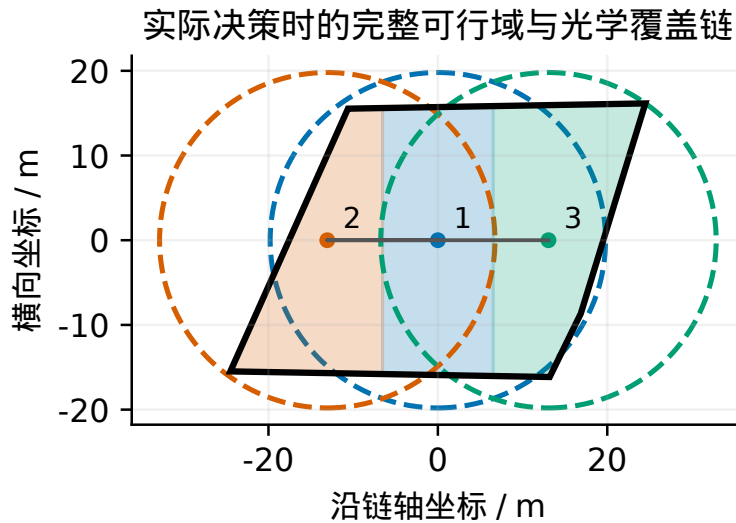
图 5 来自固定离线 Q4 案例的一次实际光学链决策。黑色边界为当时保守源域，虚线圆半径为 19.8 米，填色区为 Voronoi 责任块；数字为候选执行次序。以首点为原点、首末点连线为横轴作刚体变换，不改变覆盖关系。图中不使用源真值。
