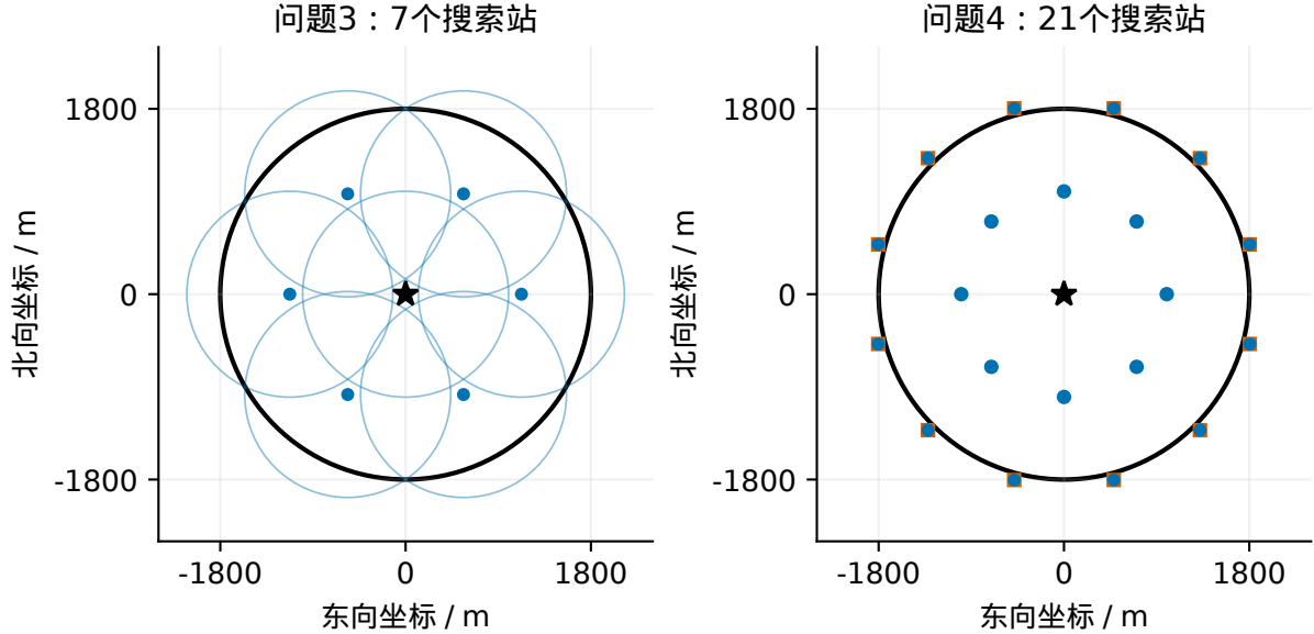
图 3 初始搜索点布局。左图中，问题三的七个 1000 米接收圆覆盖 1800 米源域，使每个全向源至少能在一站被接收。右图为问题四所用的 21 站布局。搜索点确定可发现的范围，实际访问次序随观测和清除进度调整。
