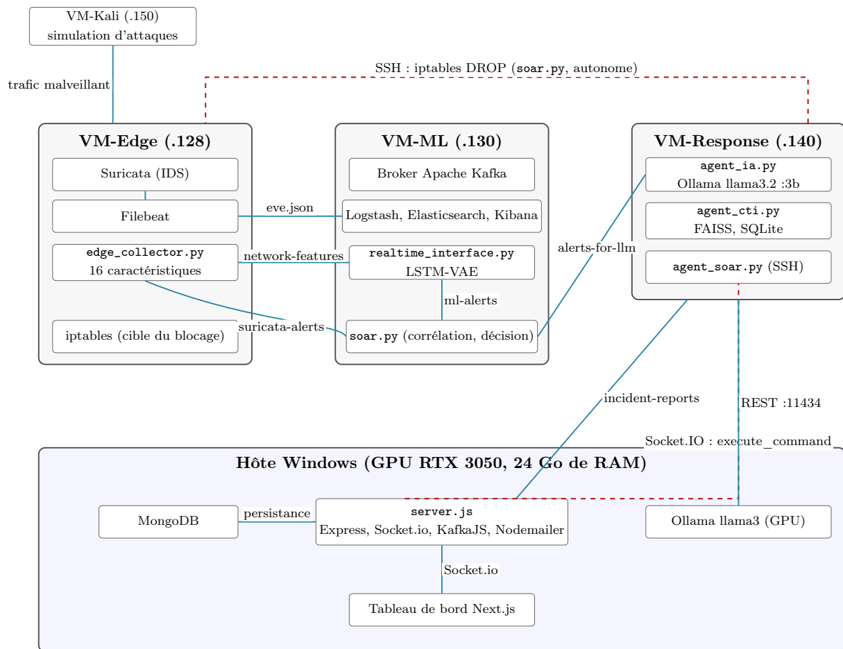
FIGURE 2.13 – Architecture de déploiement de NG-IDPS
