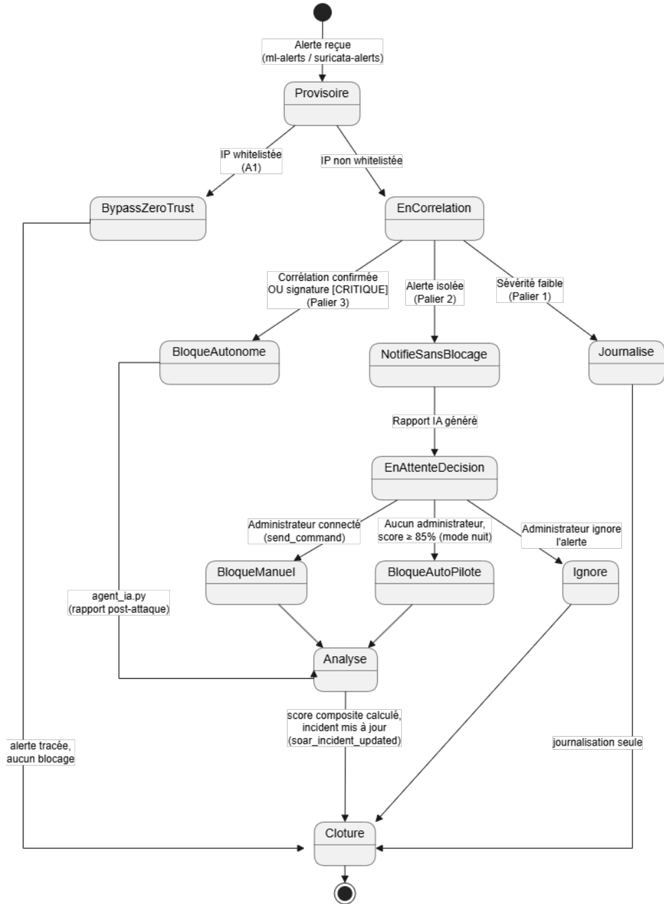
FIGURE 4.25 – Diagramme d'états d'un incident SOAR
