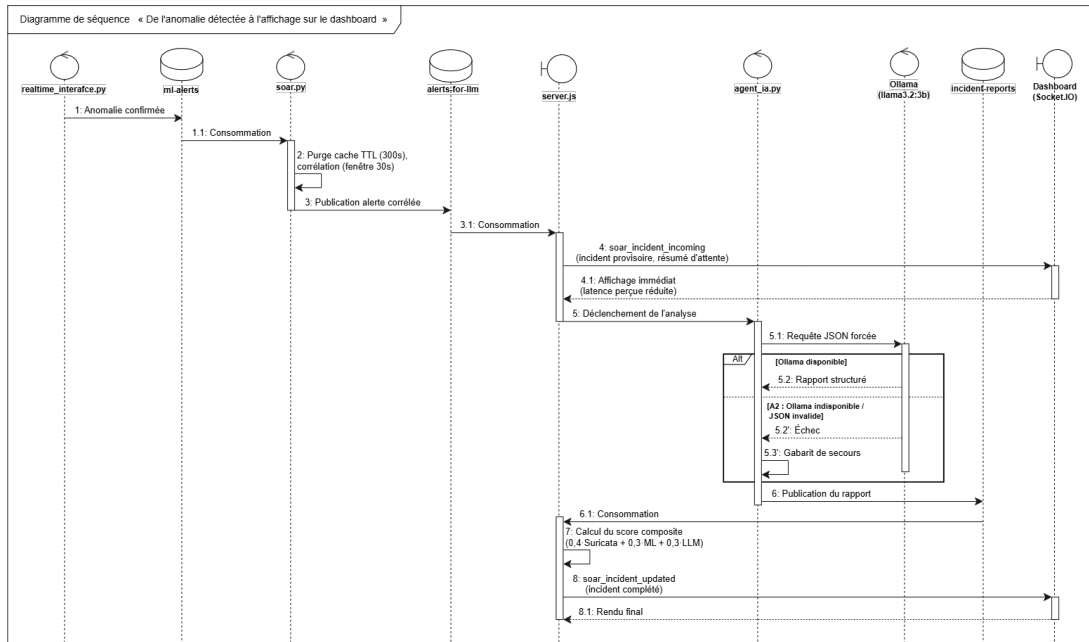
FIGURE 4.23 – Diagramme de séquence « de l'anomalie détectée à l'affichage sur le dashboard »
