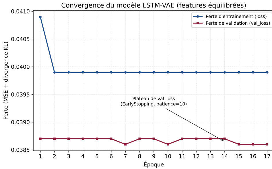
FIGURE 3.13 – Courbes de convergence algorithmique du modèle LSTM-VAE avec Early Stopping
