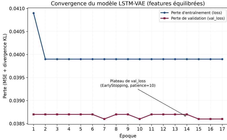
FIGURE 3.18 – Courbes de convergence algorithmique du modèle LSTM-VAE avec Early Stopping
