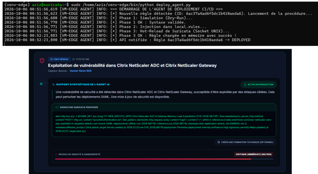
FIGURE 4.4 – Génération et validation d'une règle Suricata candidate
