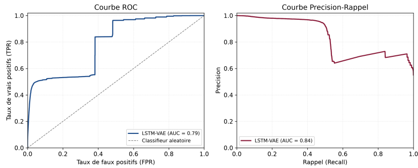
FIGURE 3.11 – Courbes ROC et Précision-Rappel sur le jeu de calibration
