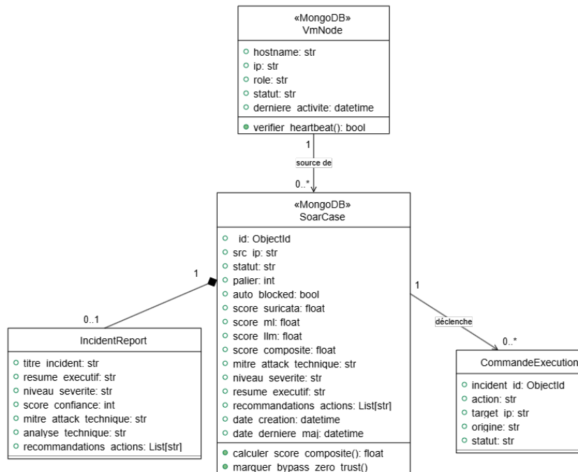
FIGURE 4.26 – Diagramme de classes du sprint 6
