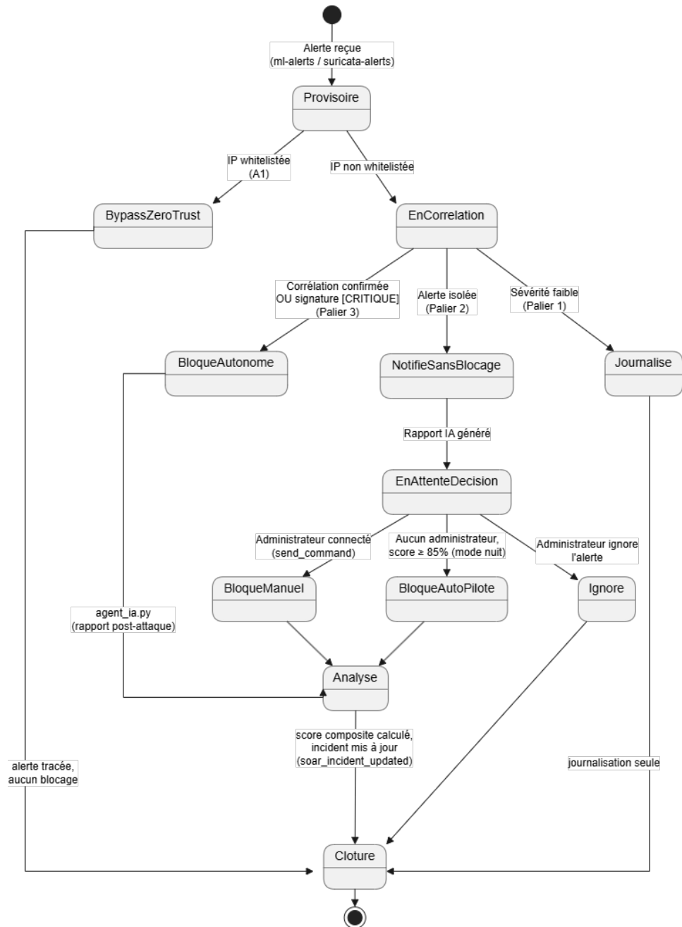
FIGURE 4.27 – Diagramme d'états d'un incident SOAR
