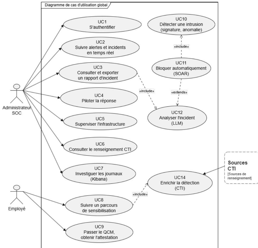
FIGURE 2.1 – Diagramme de cas d'utilisation global de NG-IDPS
