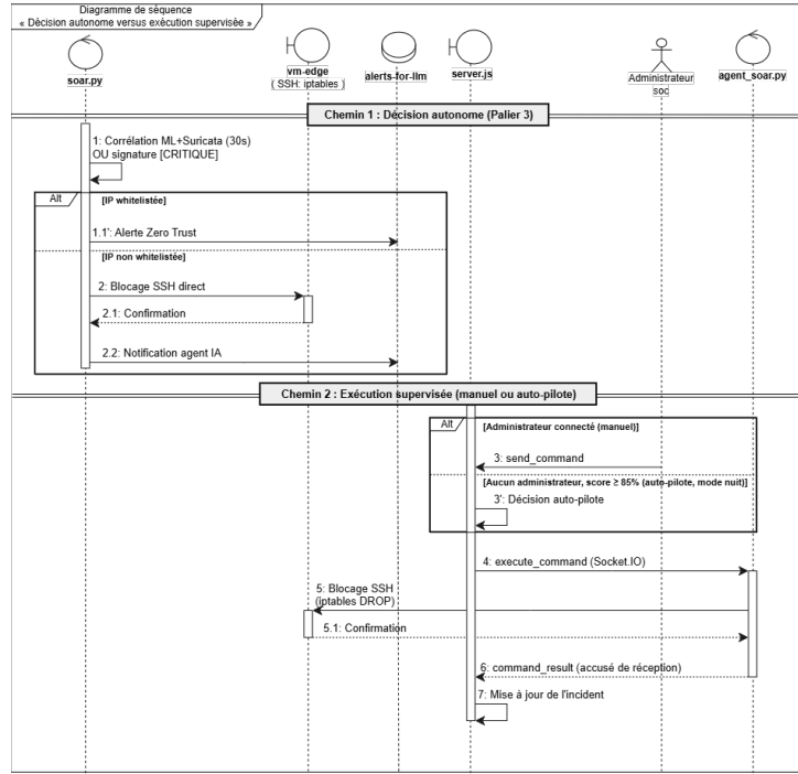
FIGURE 4.25 – Diagramme de séquence « décision autonome versus exécution supervisée »
