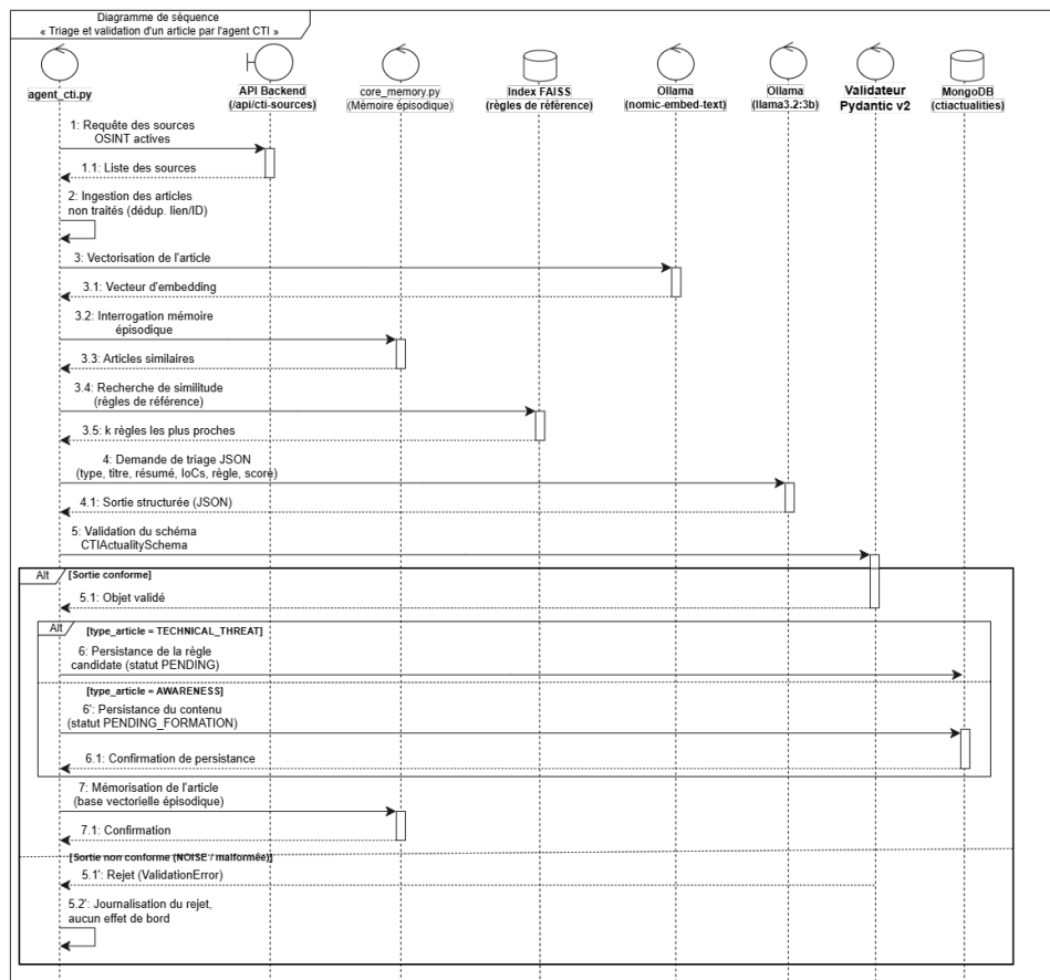
FIGURE 4.2 – Diagramme de séquence "triage et validation d'un article par l'agent CTI"
