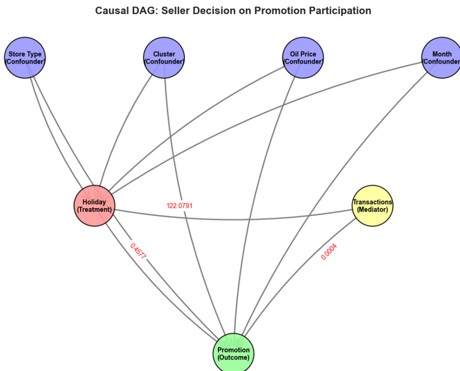
Gambar 1 DAG
