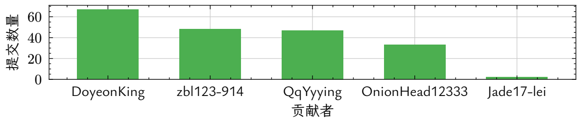
图 29 hospital_system - 贡献者提交数量统计
