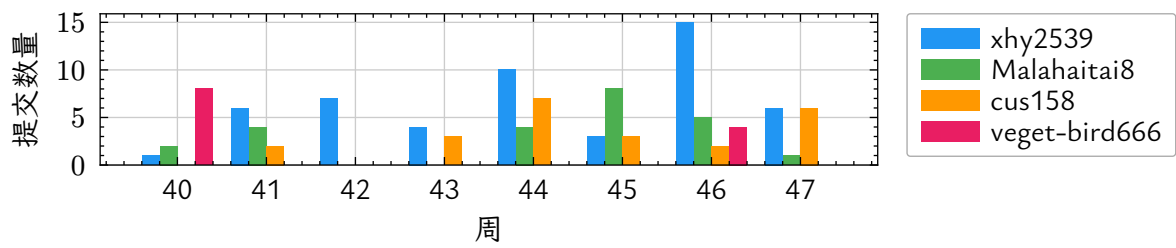
图 36 YiDianTong - 每周提交趋势（按贡献者）
