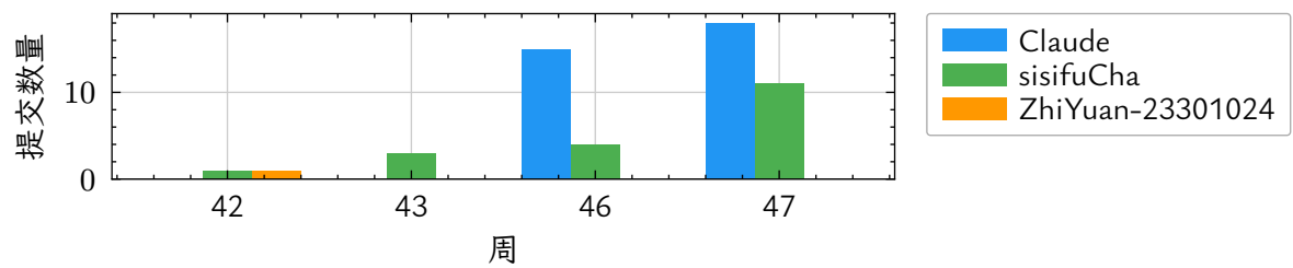
图 12 hgy-administer-frontend - 每周提交趋势 (按贡献者)
