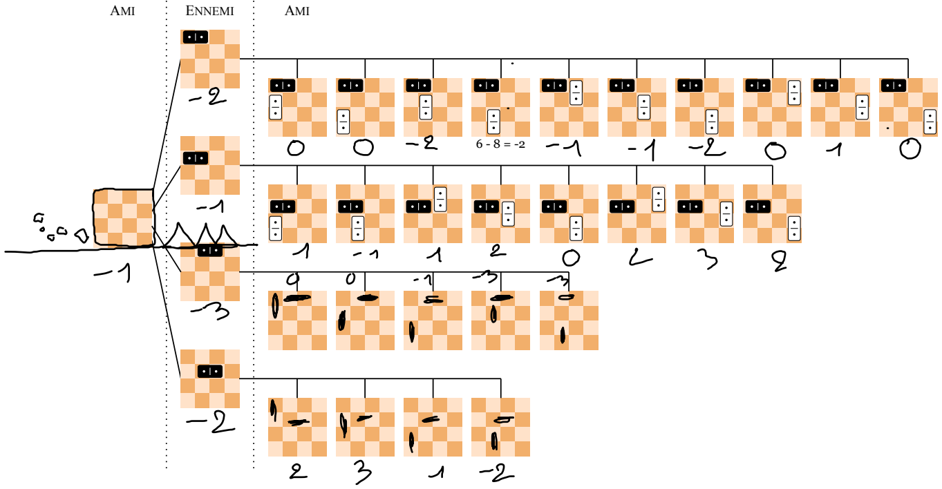
FIGURE 2 – Arbre de jeu à profondeur 2.
