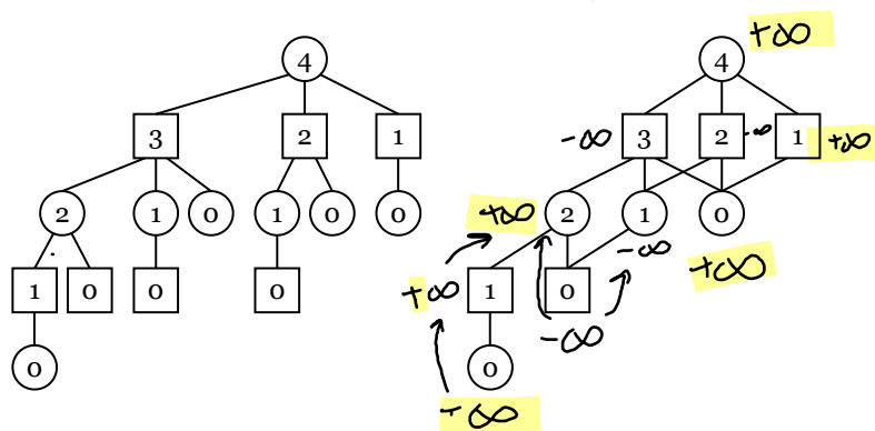
FIGURE 1 – Arbre de jeu entier pour m = 4 (à droite, écriture compact).
