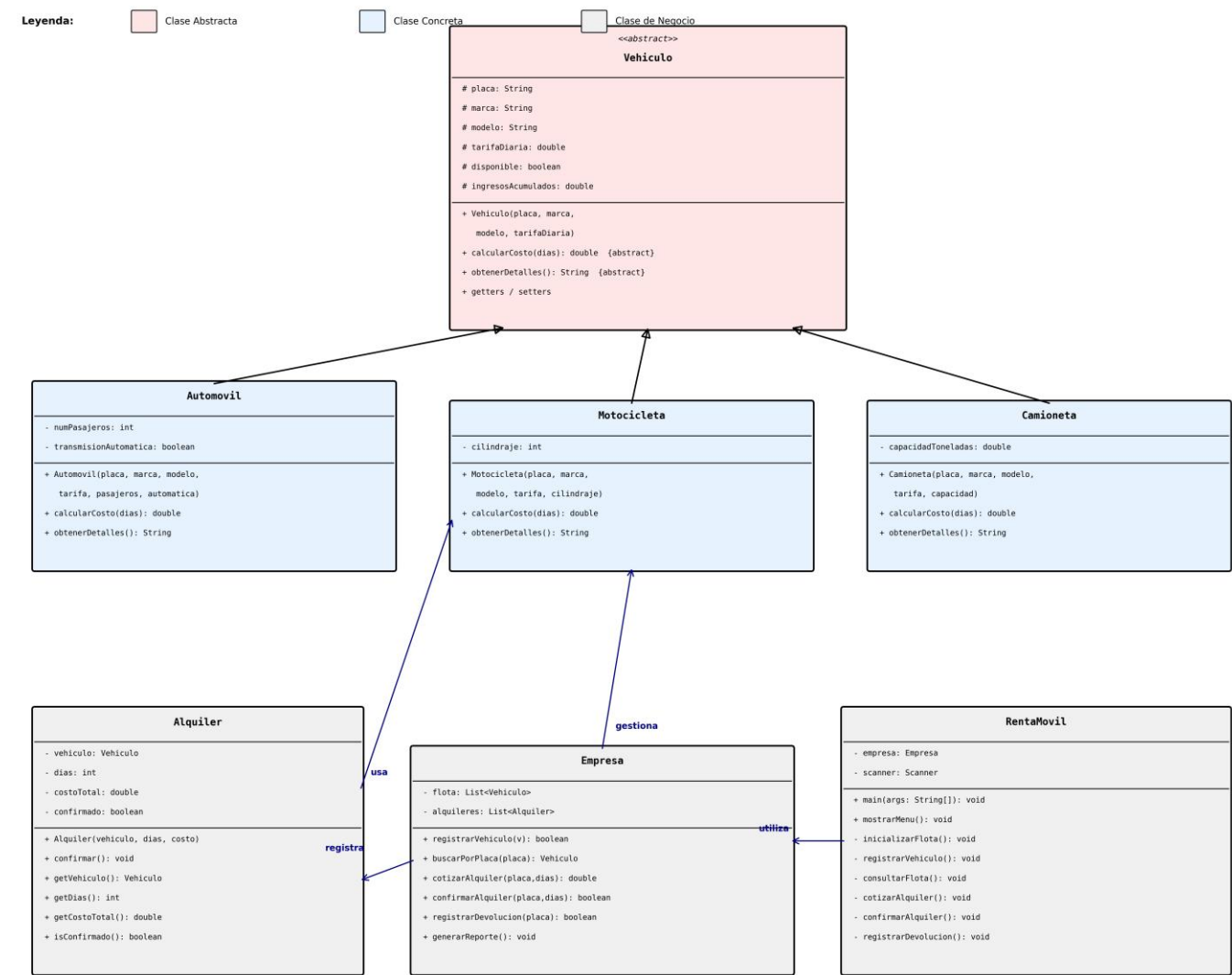
Diagrama de Clases UML - RentaMovil
