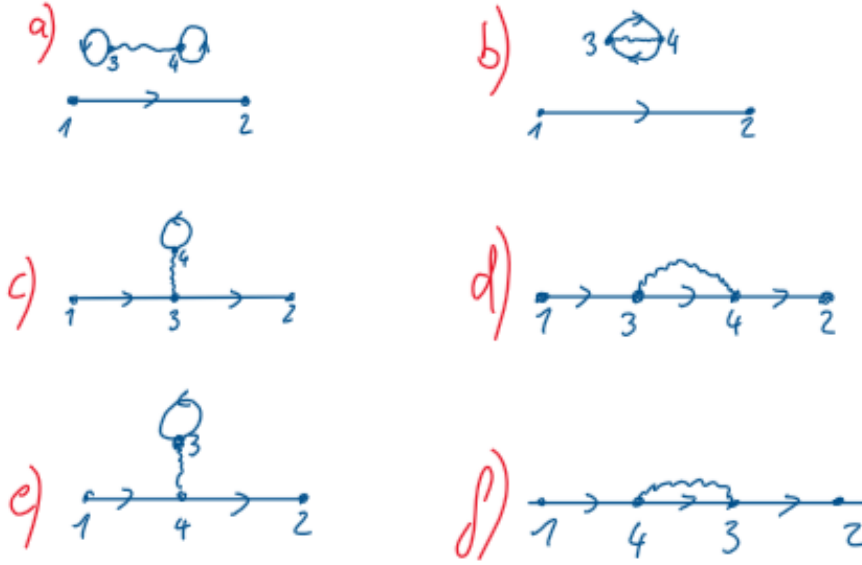
Abbildung 4: Feynman-Diagramme für die Terme a) bis f) in der Entwicklung von G^{(1)}(1, 2) .
