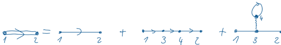
Abbildung 5: Chematische Darstellung der Feynman-Diagramme für die Störungsentwicklung von G(1,2) bis zur ersten Ordnung. Alle doppelten bzw. unnötigen wurden direkt rausgekürzt. Dadurch Fallen die Terme 1/n! und 1/2 weg. Allgemein ist mit der Wellenlinie immer i\hbar V gemeint. Deswegen fehlt der Term in dem Bild.
