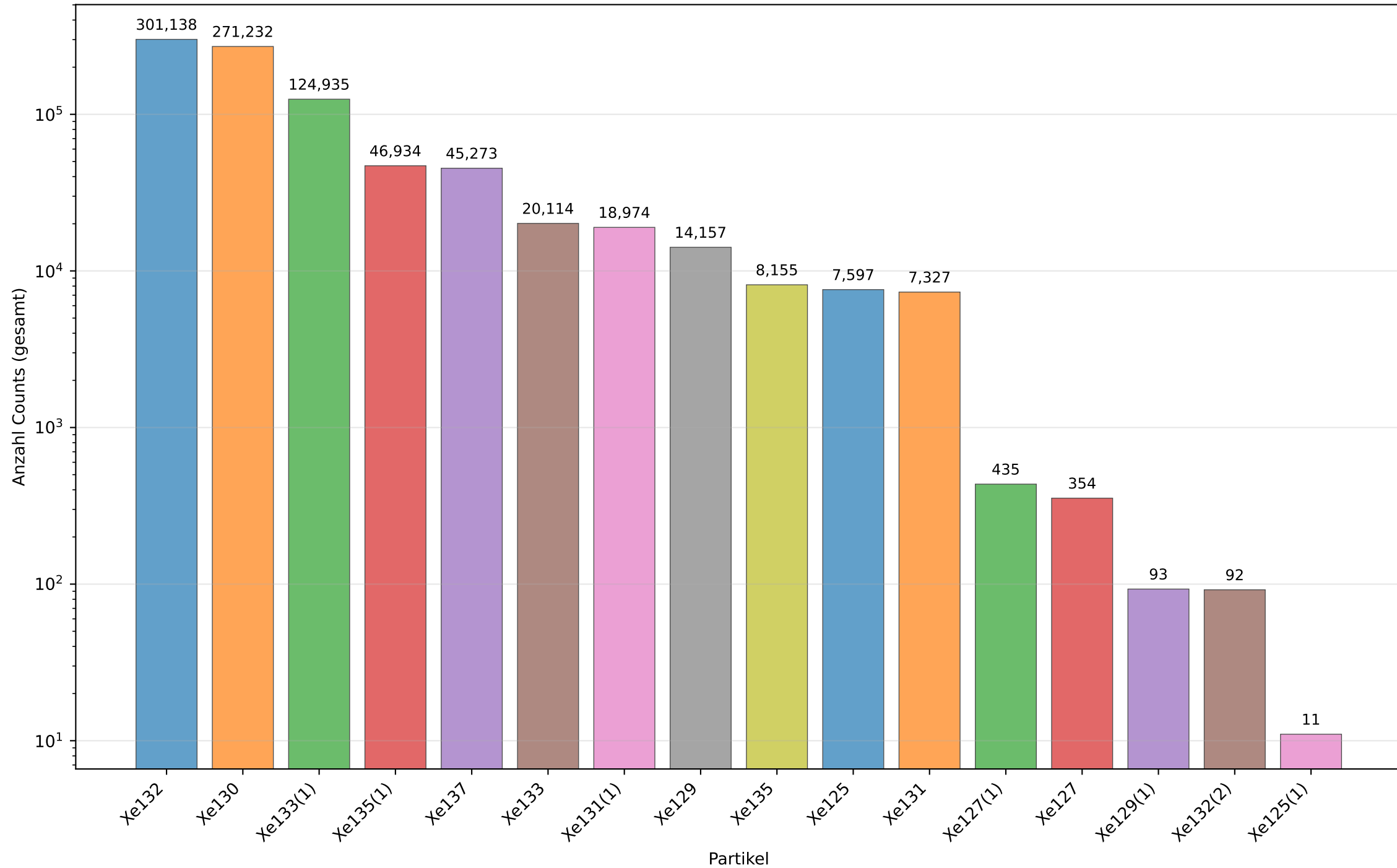
Neutron Capture Produkte in LXe - Gesamtzahlen (10cm, NoAbsorber)
