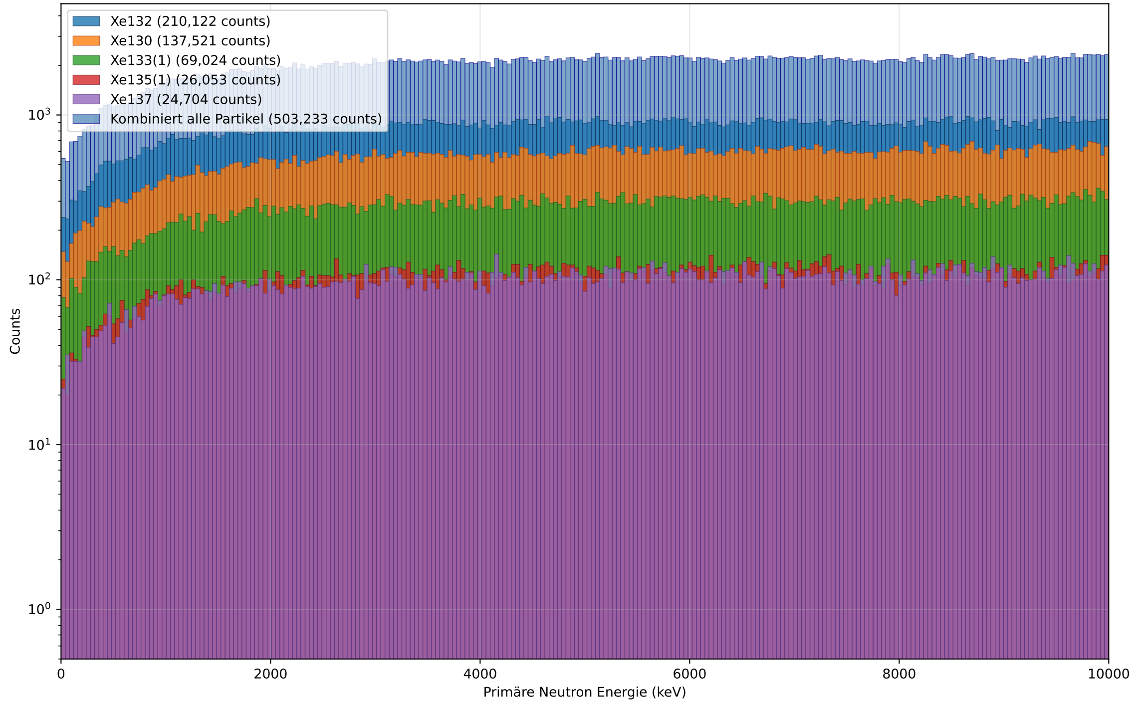
Kontroll-Plot: Neutron Capture Produkte in LXe (10cm, Polyethylen) - 16 Partikeltypen
