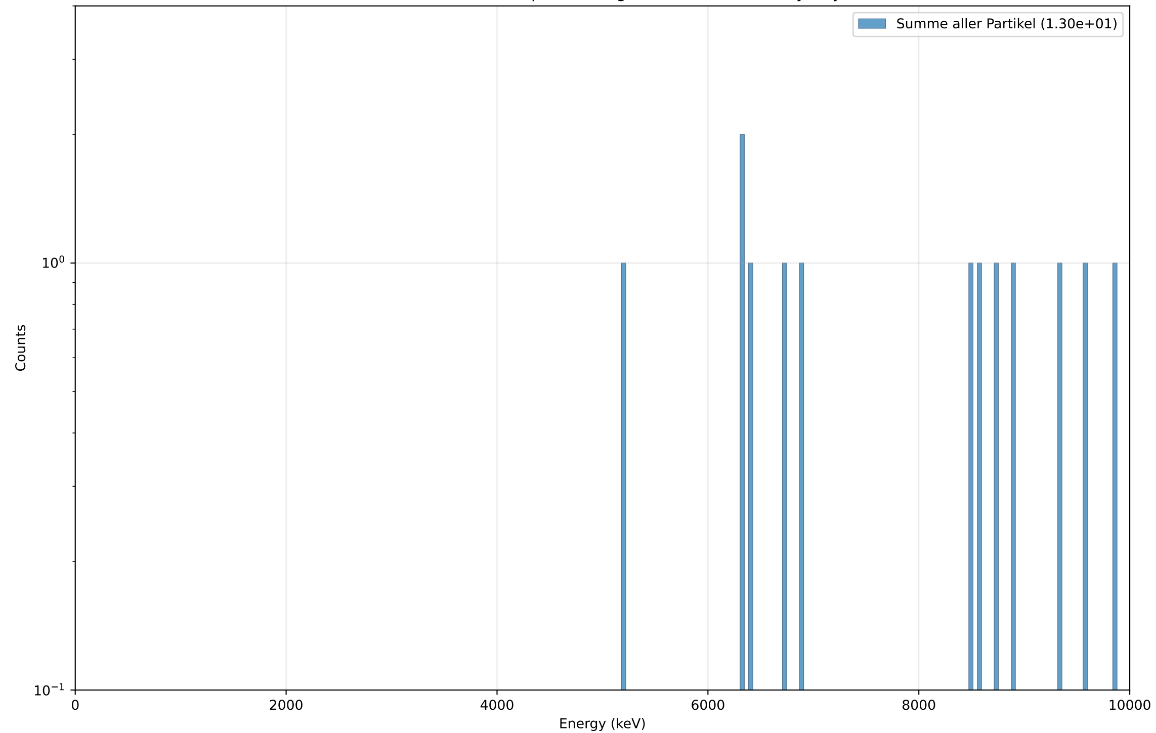
Summe aller Neutron Capture Energien in LXe (50cm, Polyethylen)
