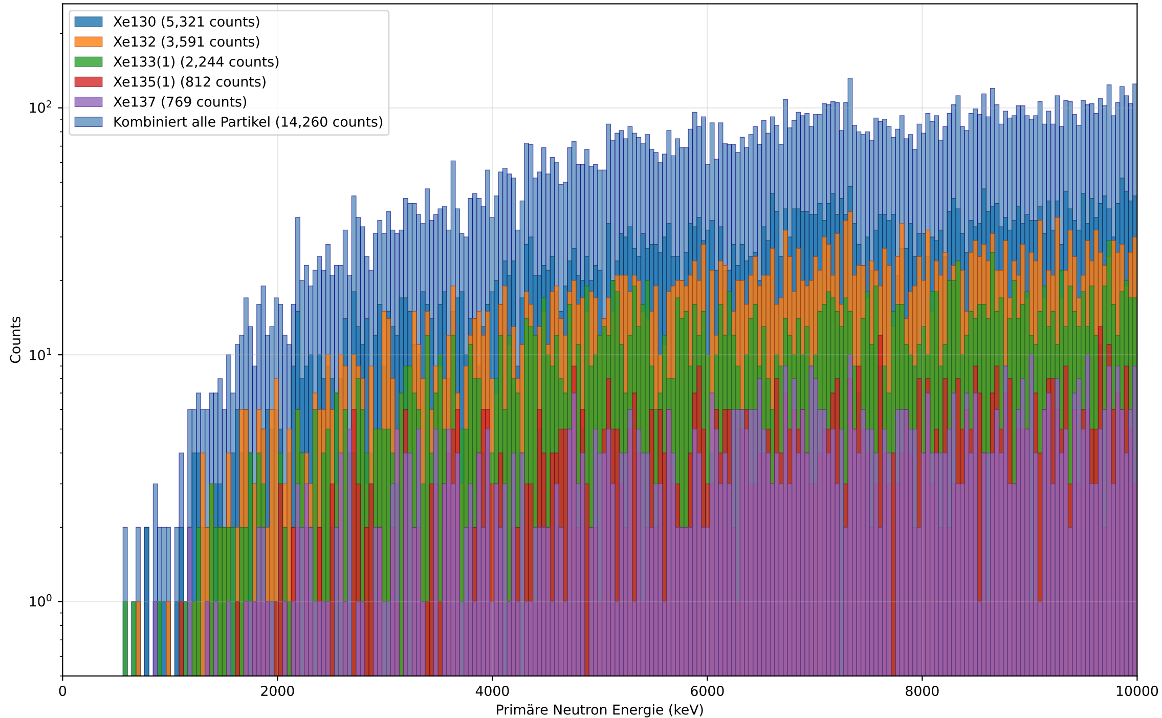
Kontroll-Plot: Neutron Capture Produkte in LXe (20cm, Polyethylen25) - 14 Partikeltypen
