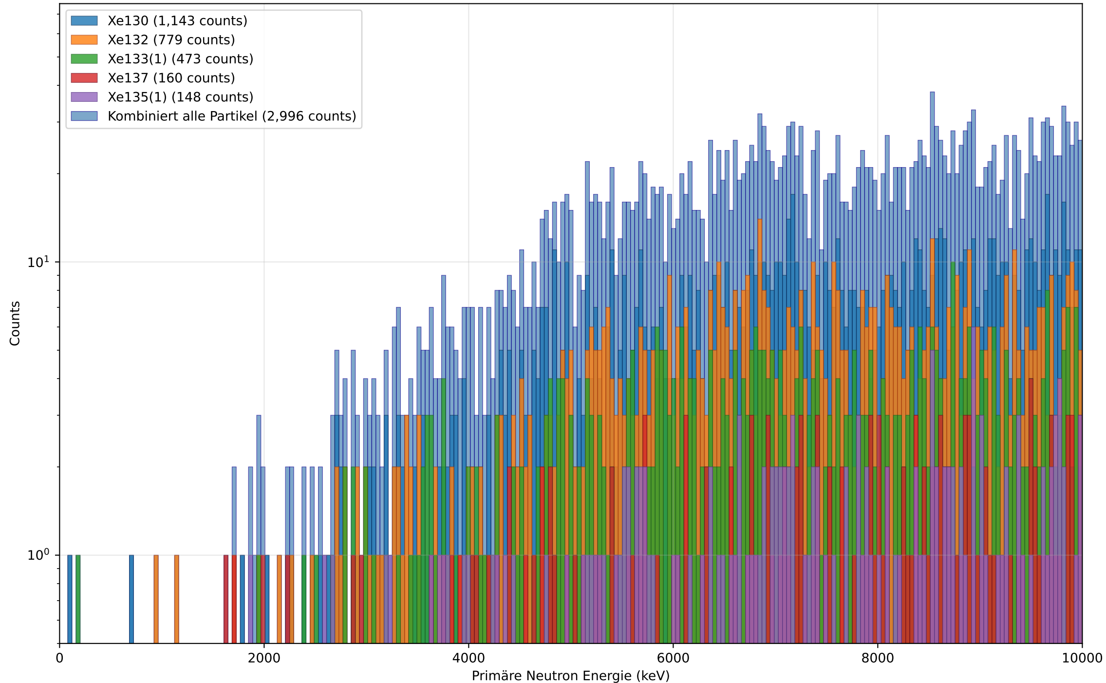
Kontroll-Plot: Neutron Capture Produkte in LXe (30cm, Polyethylen25) - 13 Partikeltypen
