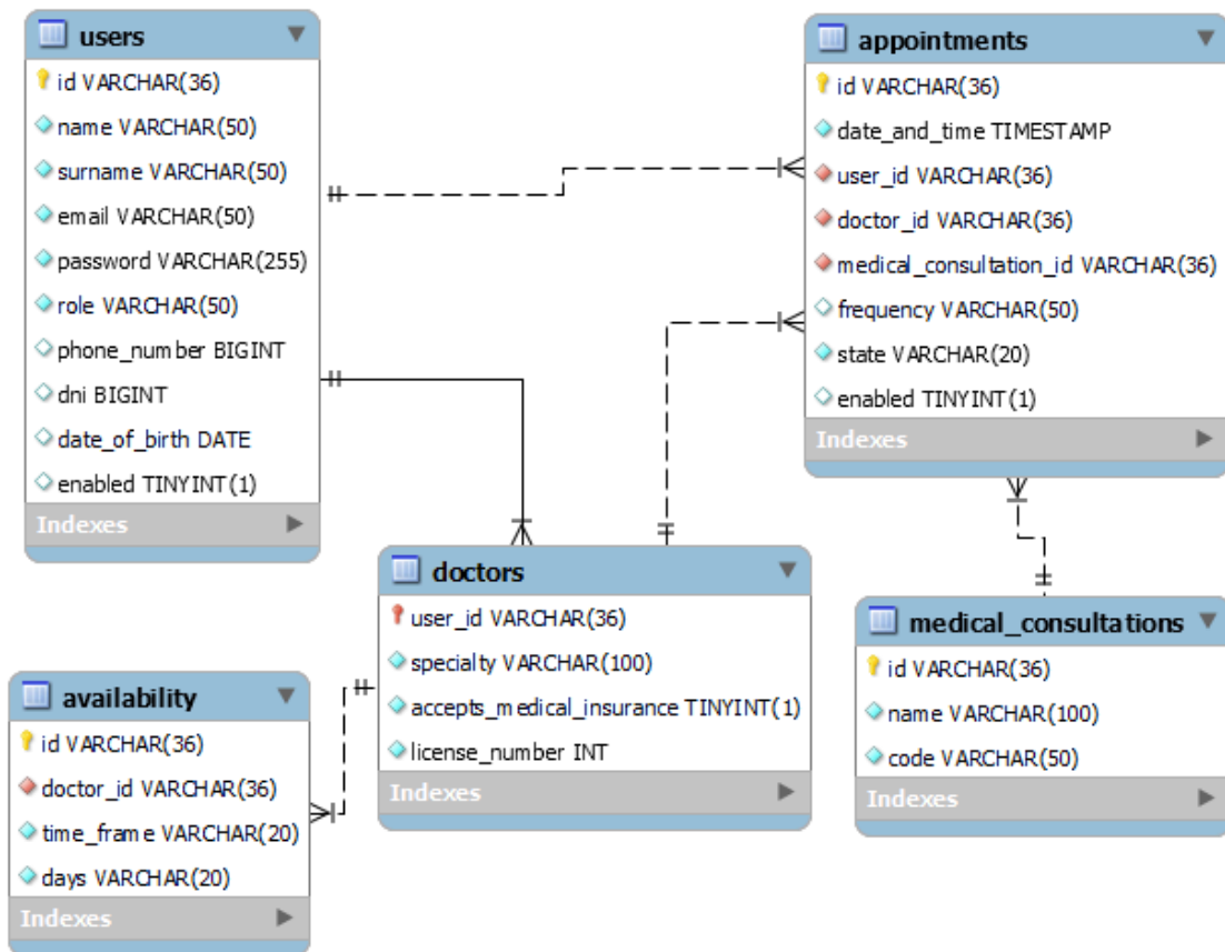
Anexo 3: Modelo relacional (Sprint 2, MVP)
