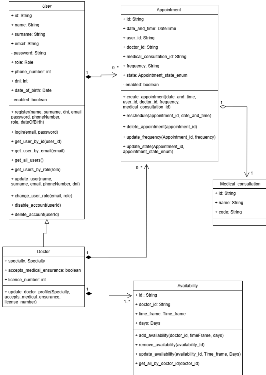
Anexo 1: Diagrama de Clases (sprint 2, MVP)
