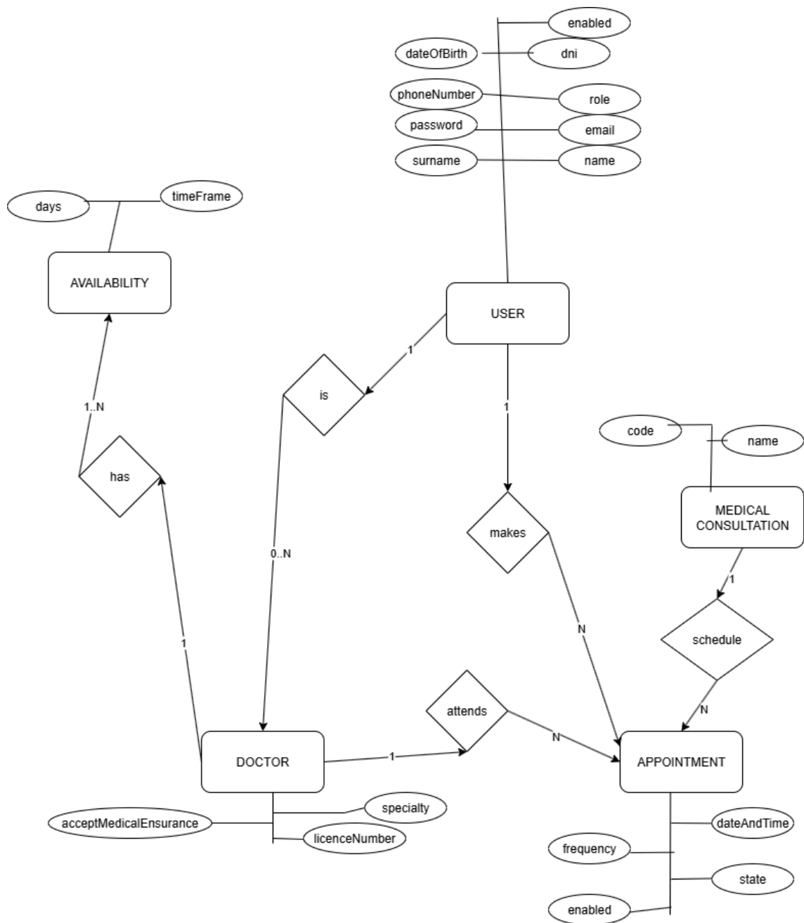
Anexo 2: Diagrama Entidad-Relación (sprint 2, MVP)
