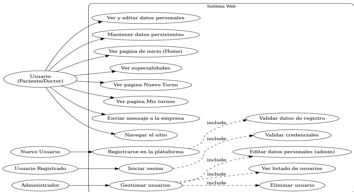
Anexo 4: Diagrama de casos de uso (Sprint 2, MVP)
