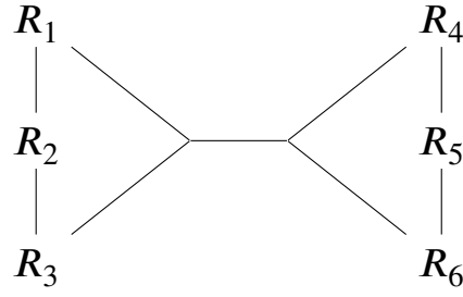
Рис. 3.1: Пример гиперграфа
