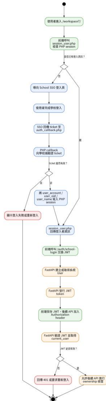
活動圖 1：使用者登入與權限驗證
