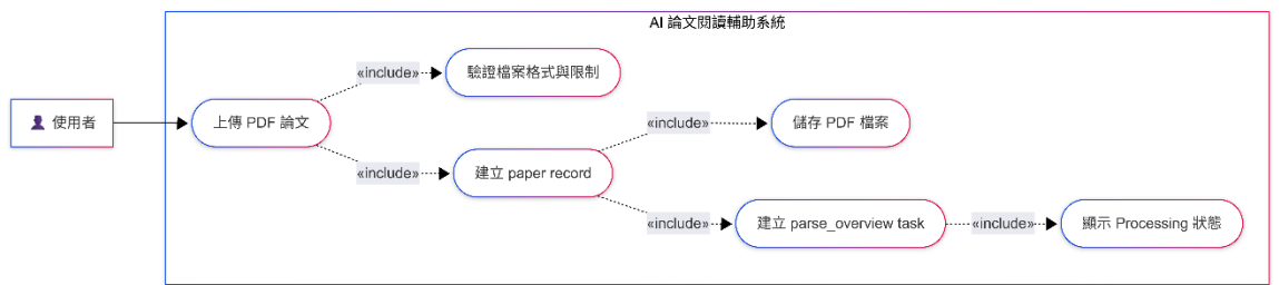
使用案例圖 2：PDF 上傳與論文建立
