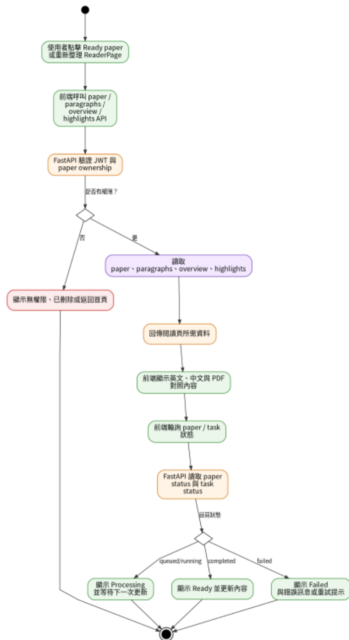
活動圖 4：ReaderPage 閱讀與任務狀態回饋
