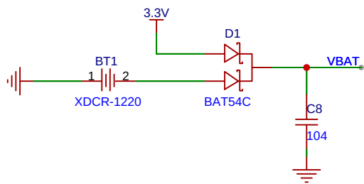
RTC时钟电池
