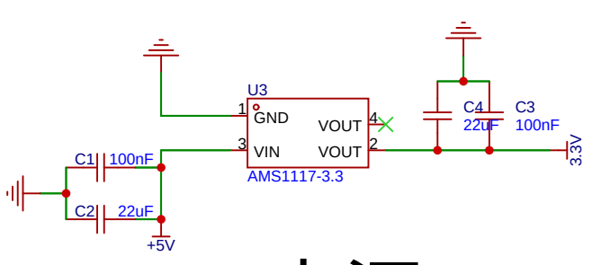
电源
