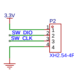
SWD
