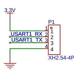
串口1
