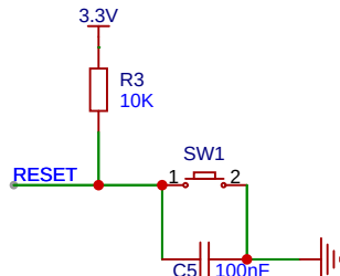
复位电路
