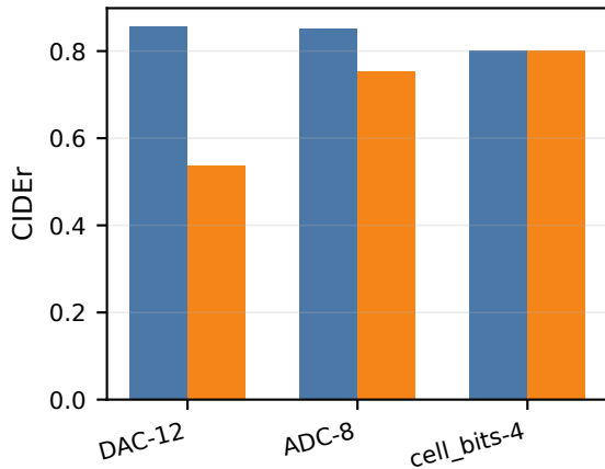
CIDEr gap
