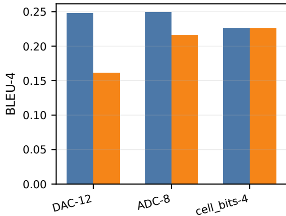
BLEU-4 gap
