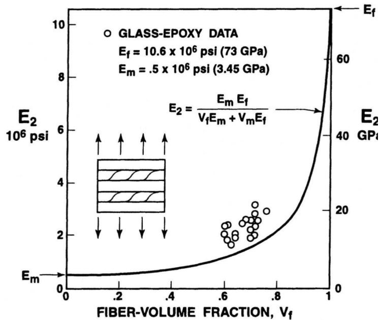
Figur 4.3: Forudsagt og målt E_2
