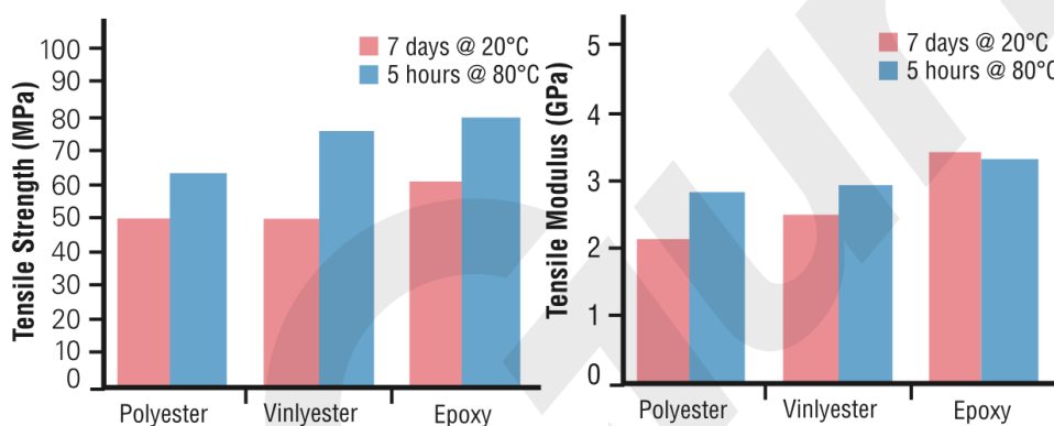
Figur 3.4: Sammenligning af resinstyrke og -stivhed, reproduceret fra (Gurit 2017, fig. 22).
