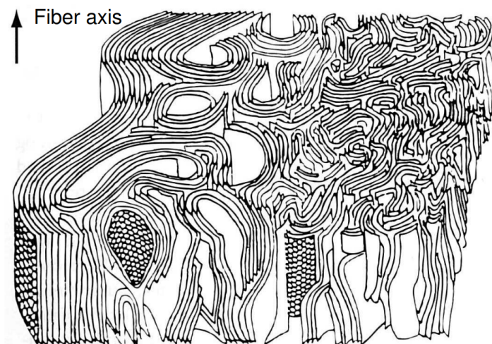
Figur 2.2: Schematisk repræsentation af strukturen af en kulfiber. Reproduceret fra (Hull og Clyne 2007, Fig. 2.1), originalt fra Benett og Johnson 1978.
