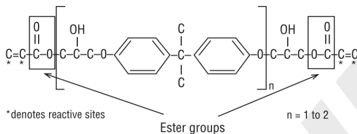
Figur 3.2: Idealiseret kemisk struktur for en typisk epoxy-baseret vinylester, reproduceret fra (Gurit 2017, fig. 16).
