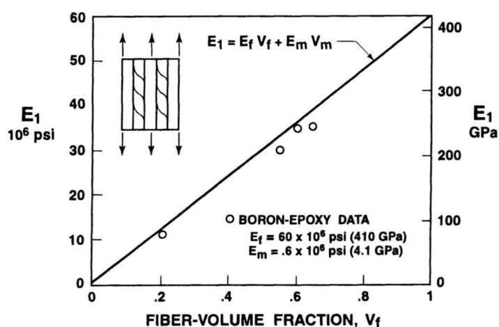
Figur 4.2: Variation i E_1 som følge af ændring af fibervolumenfraktion
