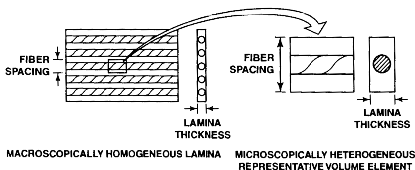
Figur 4.1: Repræsentativt volumenelement – Lamina med unidirektionelle fibre, reproduceret fra (Jones 2021, fig. 3-2).
