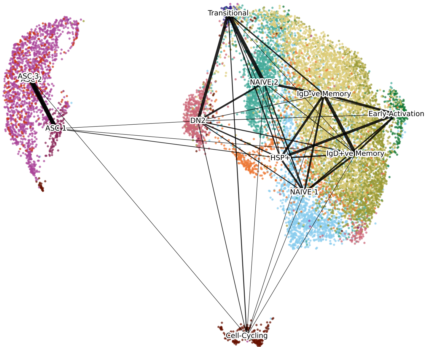
PAGA connectivity overlaid on Seurat UMAP
