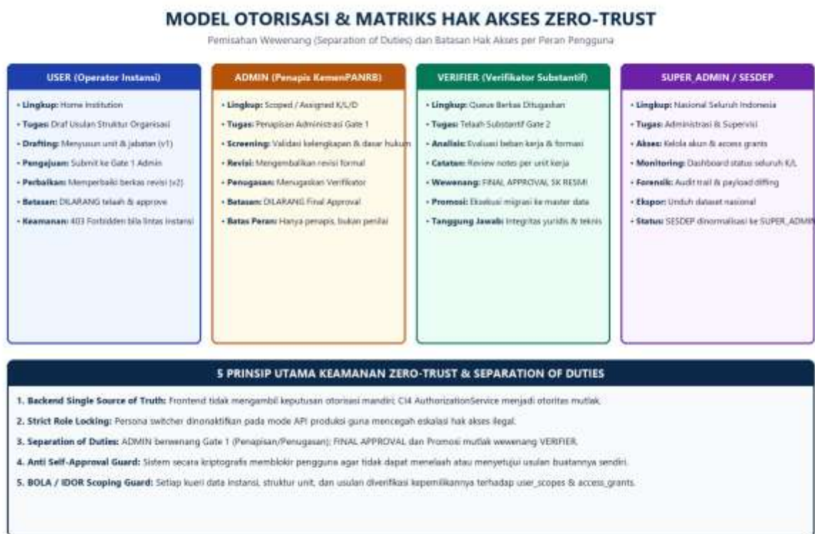
Gambar 2: Model Otorisasi dan Matriks Hak Akses Zero-Trust SIGMA-K
