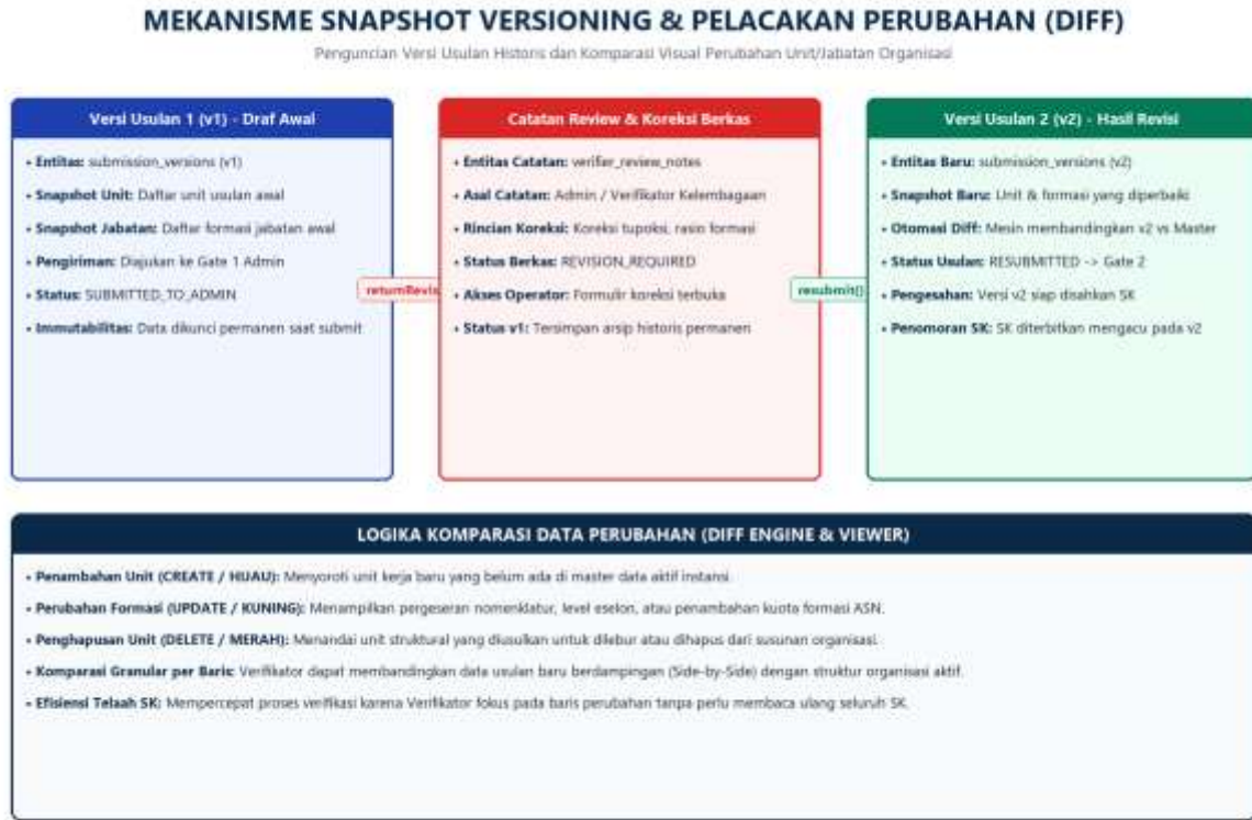
Gambar 8: Mekanisme Snapshot Versioning dan Pelacakan Perubahan Data (Diff Flow)
