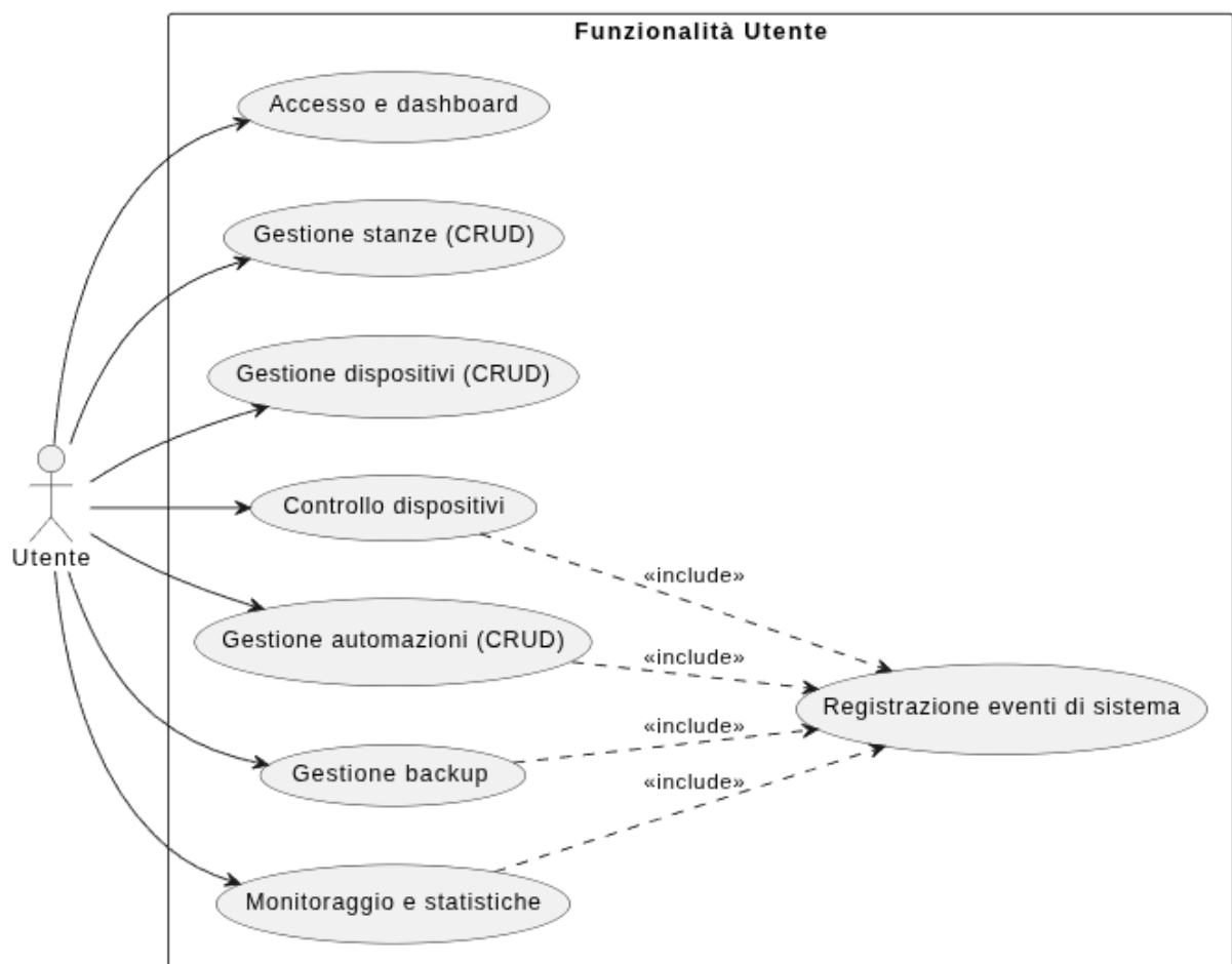
Figure 2: Gestione utilizzatore
