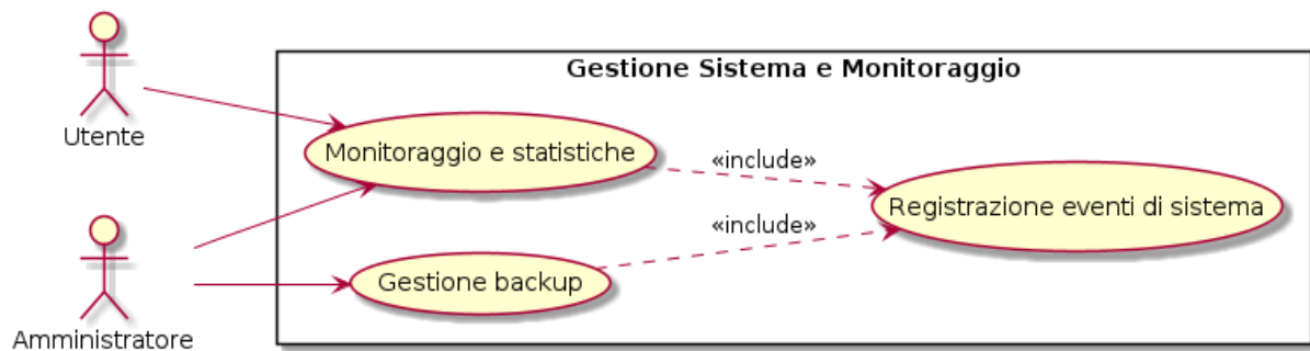
Figure 4: Gestione sistema
