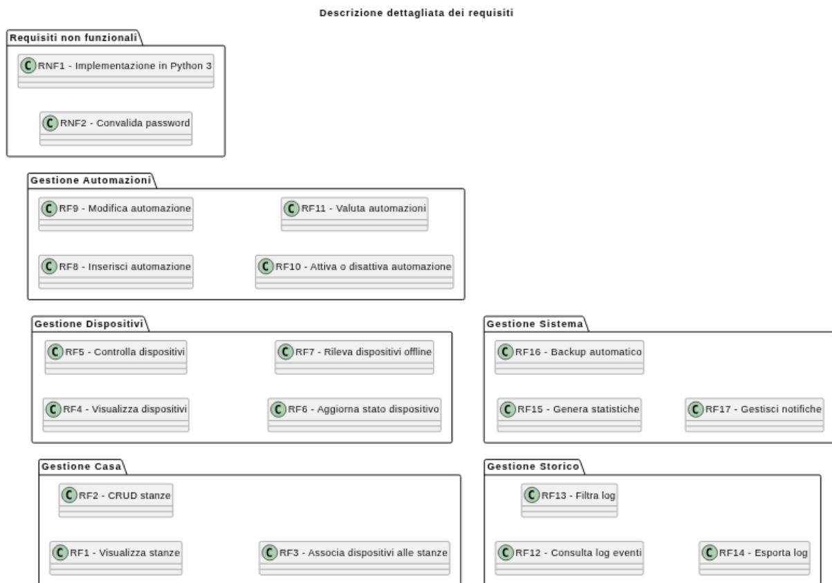
Figure 5: Dettaglio requisiti
