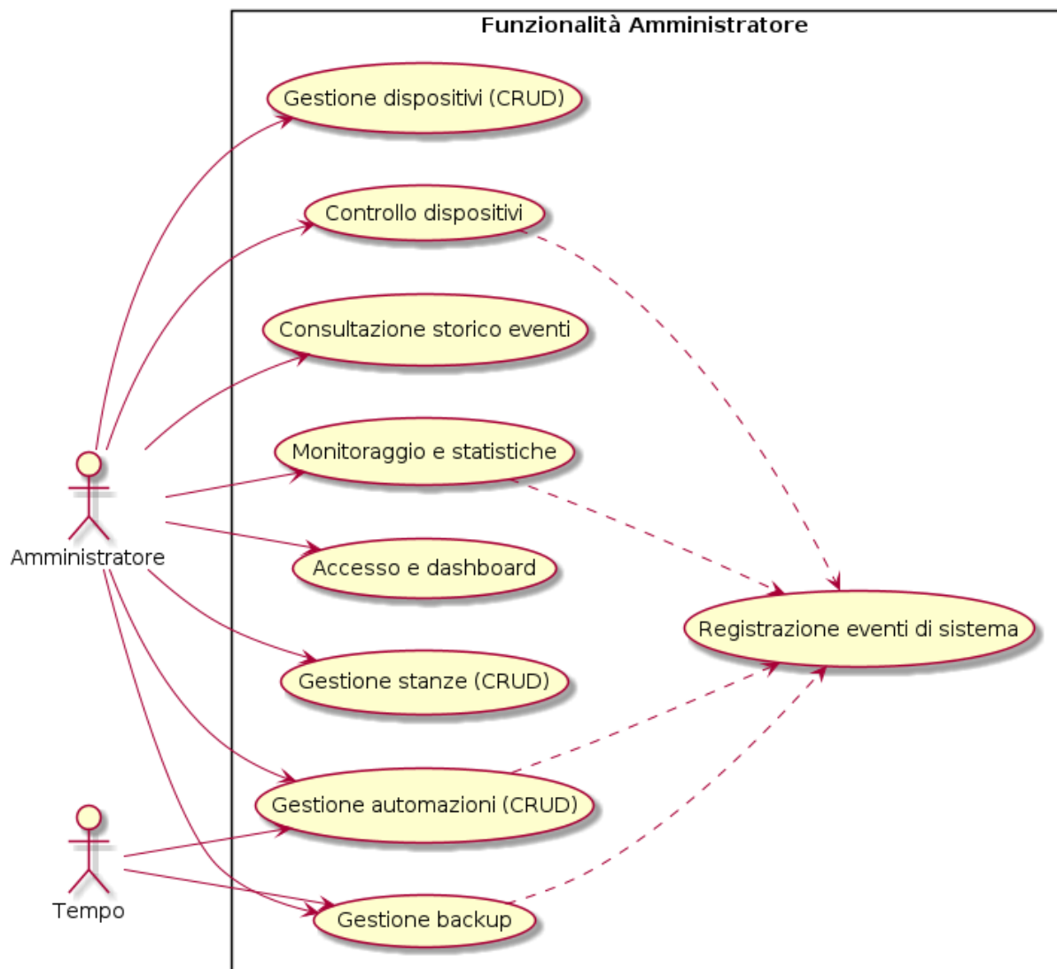
Figure 3: Gestione amministratore
