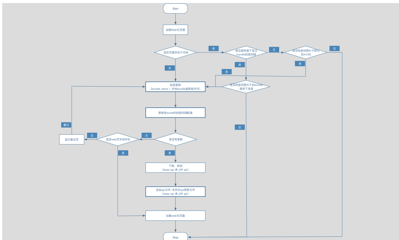
ajx-web_flowchar
