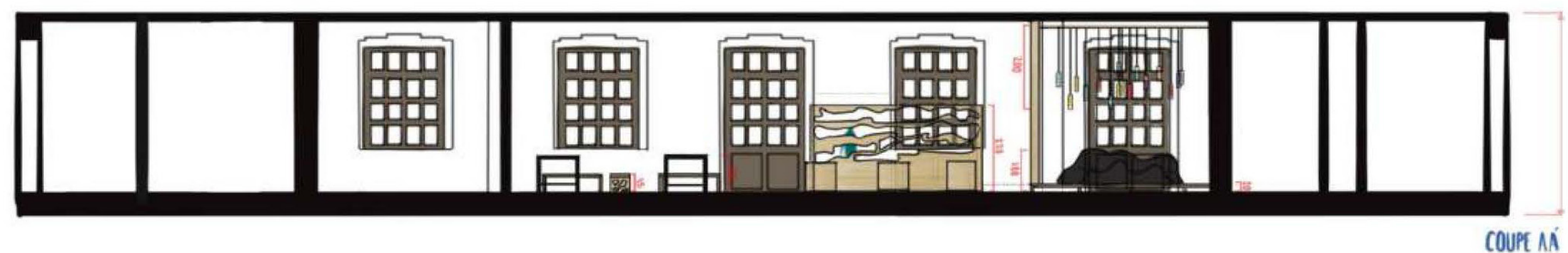
COUPE LONGITUDINALE
