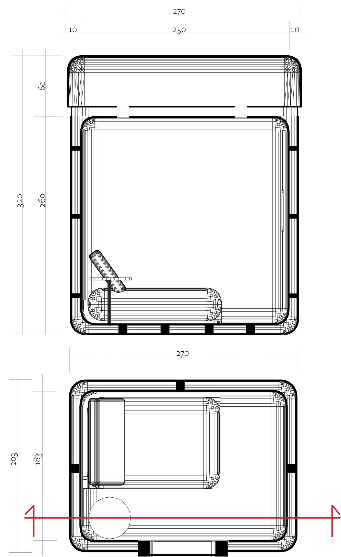
COUPE & PLAN - CAPSULE 01
