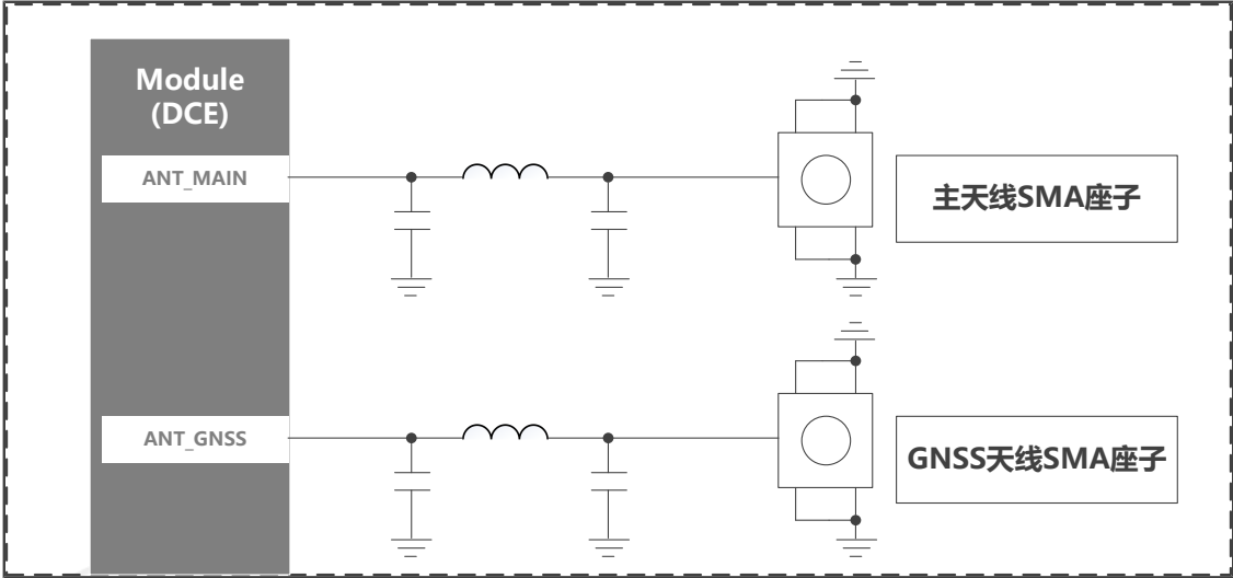
Figure 20. 模组天线接口示意图
