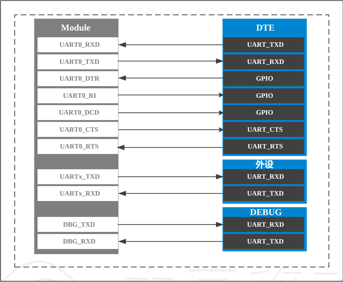
Figure 19. UART接口示意图
