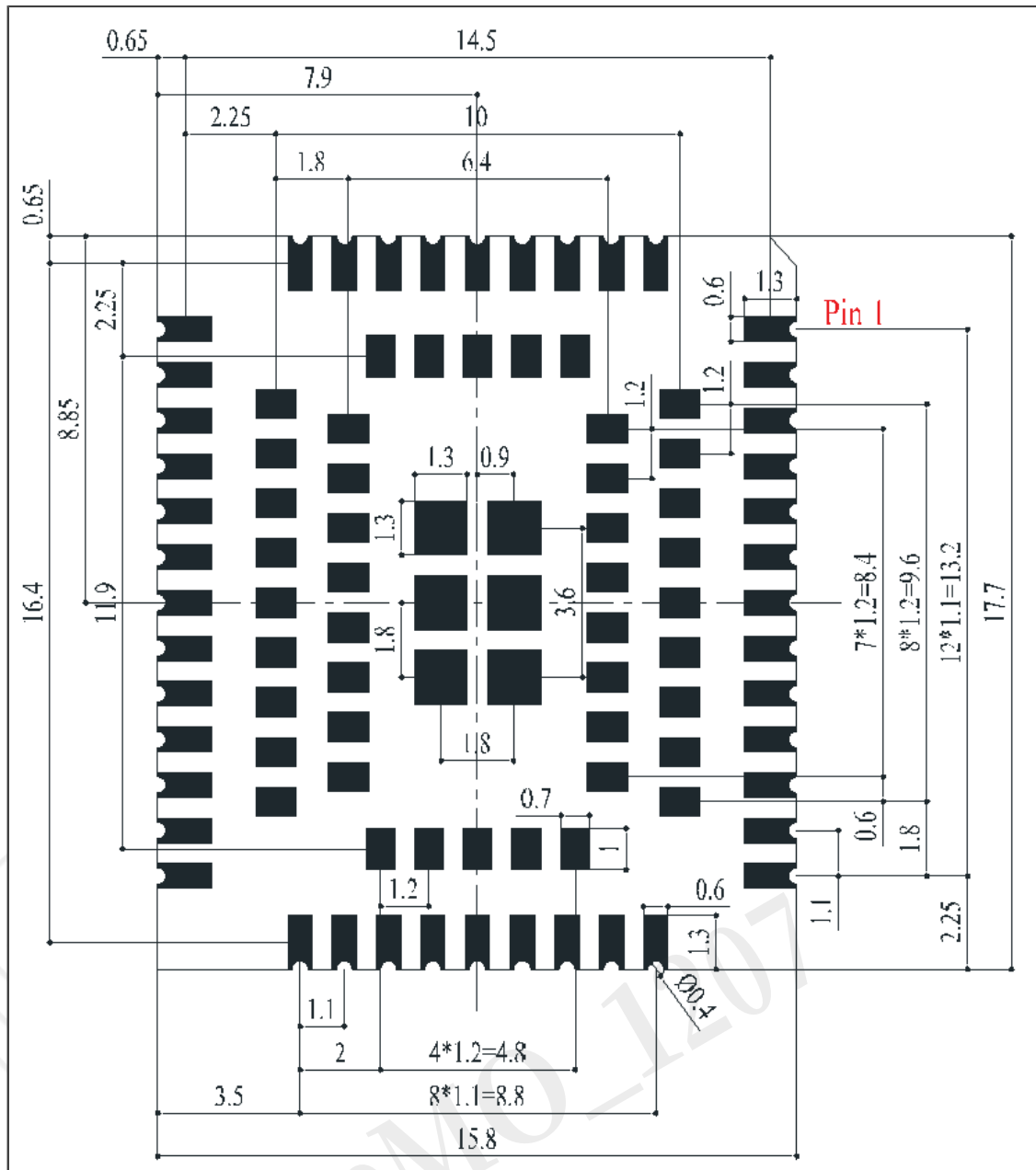
Figure 22. ML307S/ML307A-D底视图 (单位: mm)
