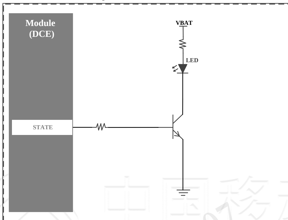
Figure 12. 模组状态接口示意图
