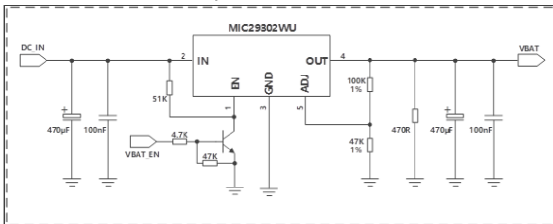
Figure 7. 供电输入参考设计
