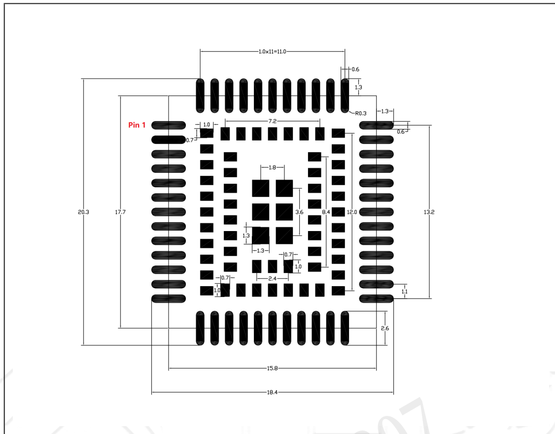
Figure 24. PCB焊盘兼容尺寸 (单位: mm)
