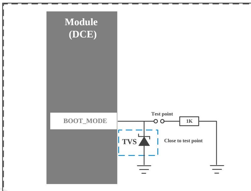
Figure 13. BOOT_MODE接口示意图
