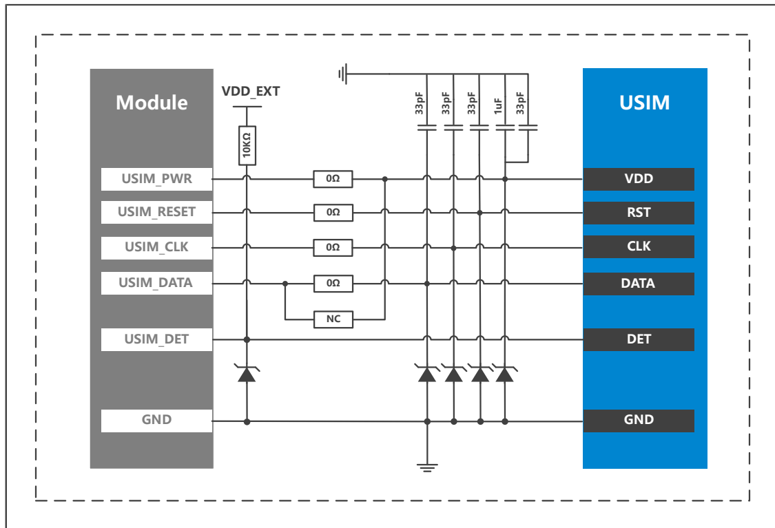
Figure 17. ML307R USIM接口示意图
