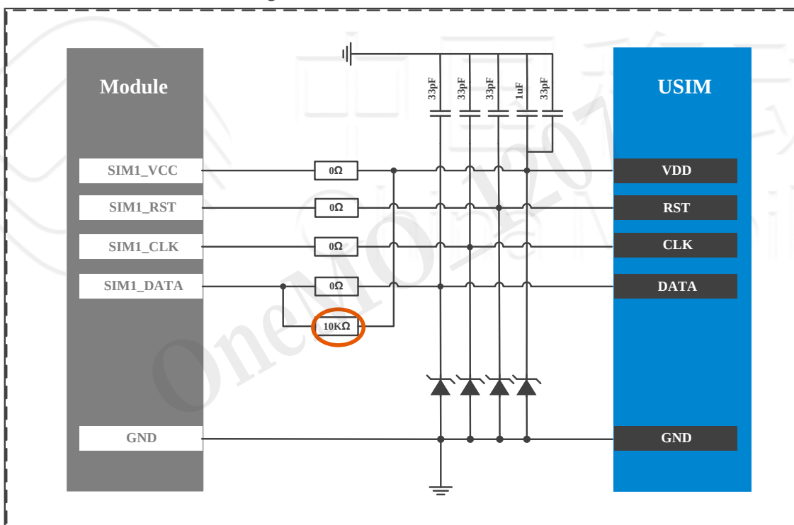
Figure 16. ML307A SIM1接口示意图
