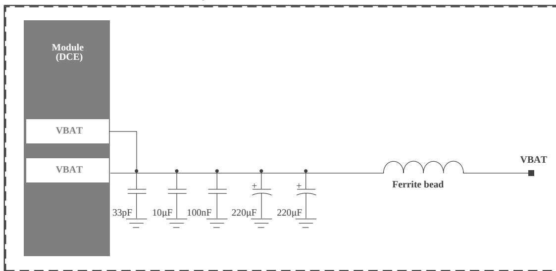
Figure 6. 模组供电电路参考设计
