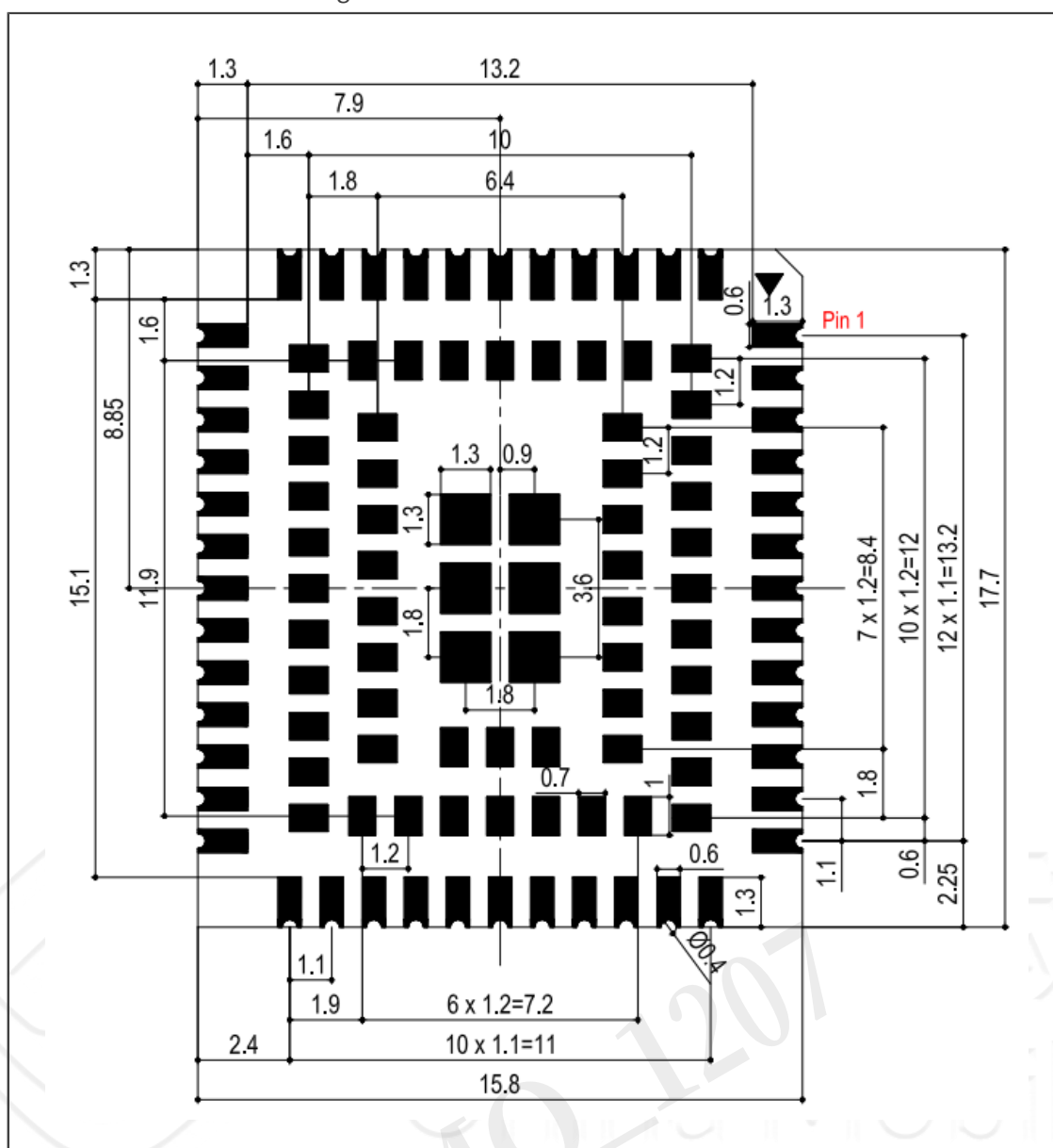
Figure 23. M307R底视图 ( 单位: mm )
