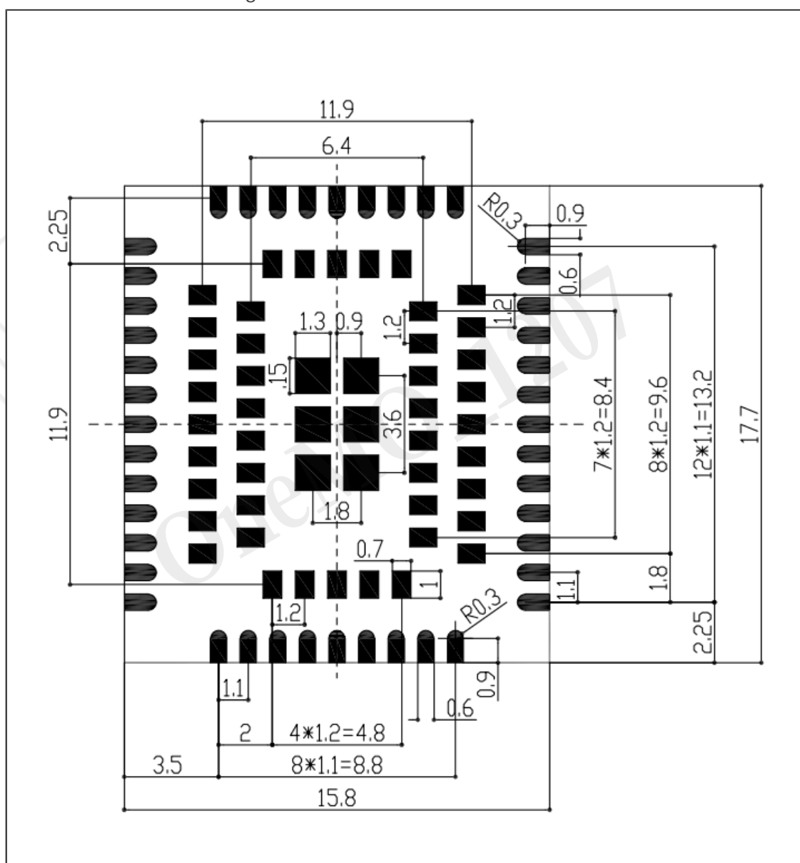
Figure 21. M307A-G底视图 (单位: mm)
