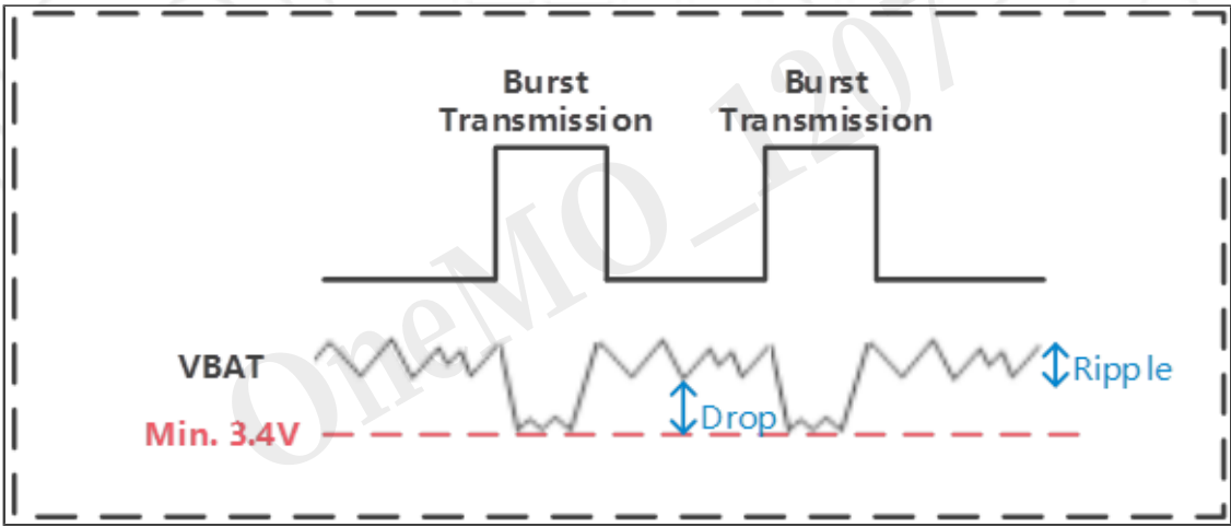
Figure 5. 突发传输电源要求
