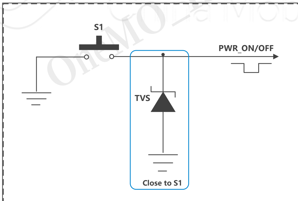
Figure 9. 按键开关机参考电路
