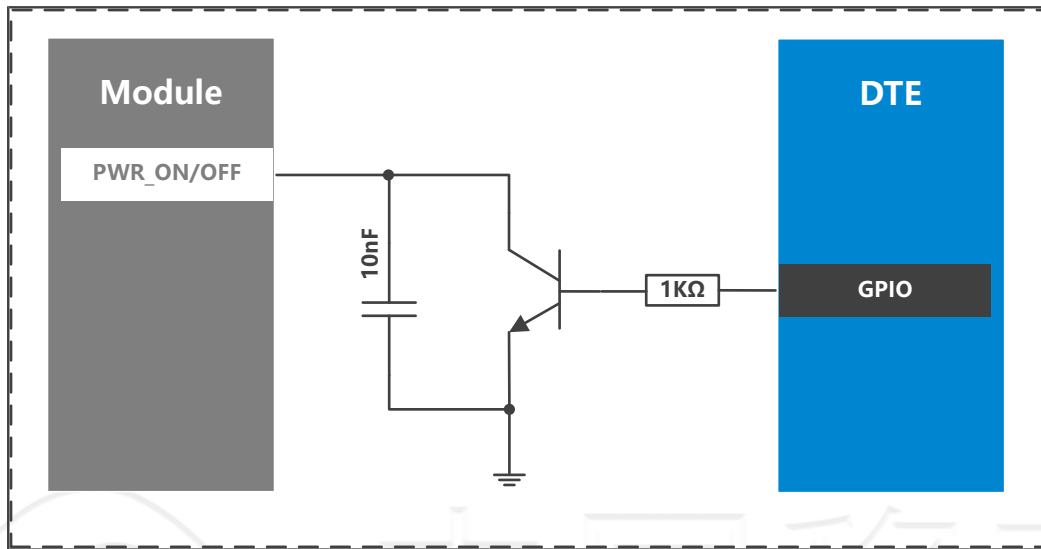
Figure 8. 开集驱动开关机参考电路
