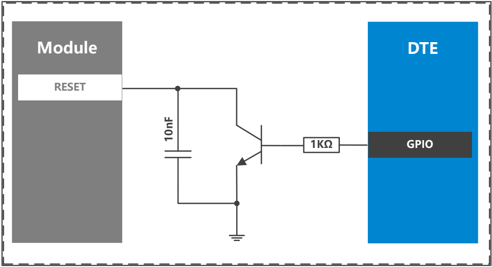
Figure 10. 模组复位参考电路
