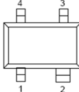
SOT343(SC-82)
