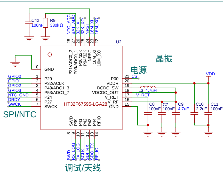
主控BLE-HT32F67595
