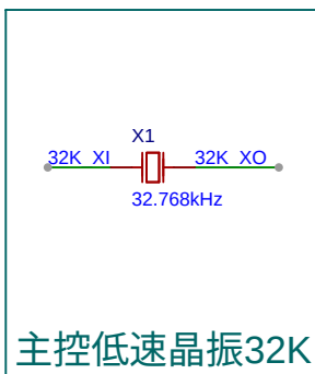
主控BLE-HT32F67595
