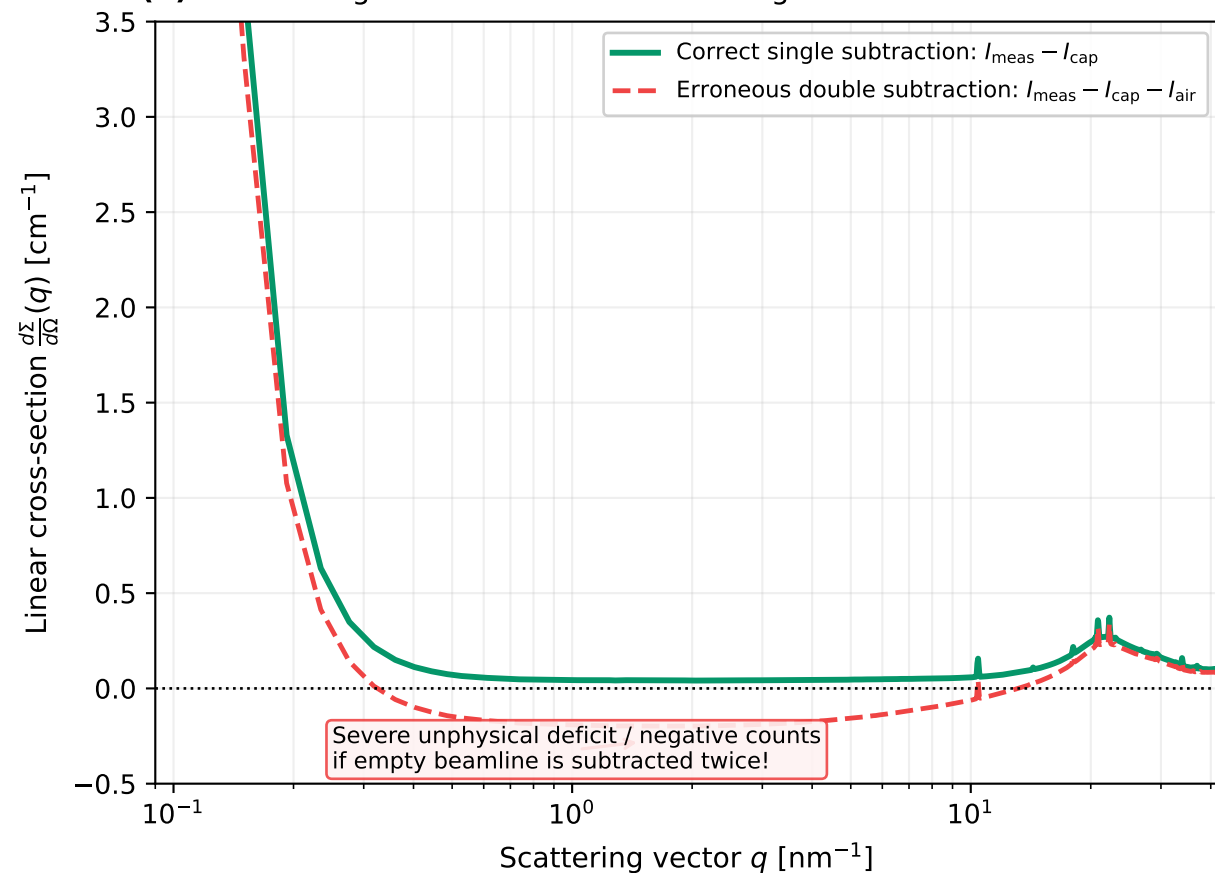
(d) Methodological demonstration: avoiding erroneous double subtraction
