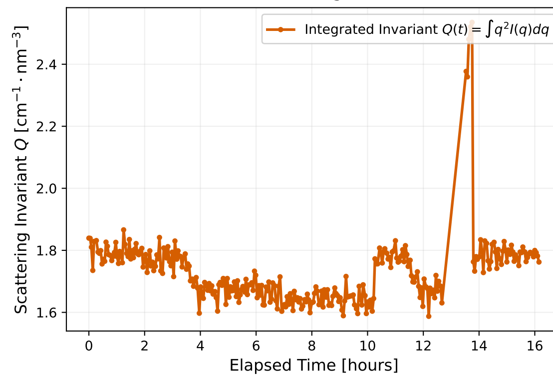
(d) Structural Scattering Invariant vs Time
