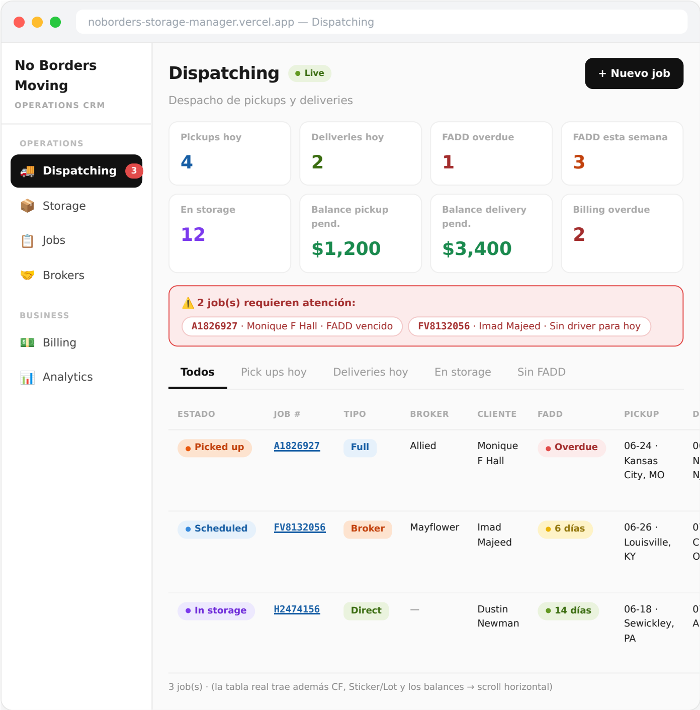
Pantalla de Dispatching: métricas arriba, banner de alertas, sub-pestañas y la tabla de jobs con sus acciones.
