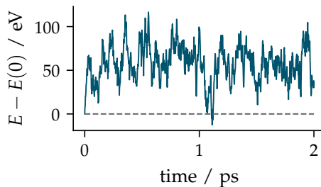
(d) wrapped bonds
