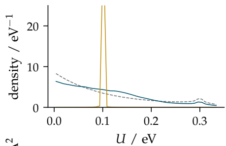
(d) one atom, one thermostat
